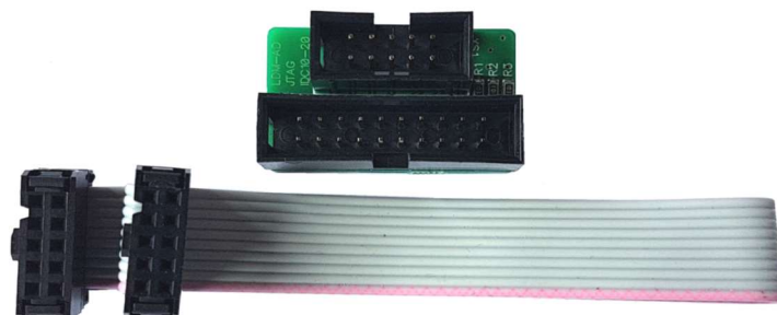
Рисунок 2. Вид переходника LDM-AD-JTAG-IDC10-20 для подключения программатора ULINK2
