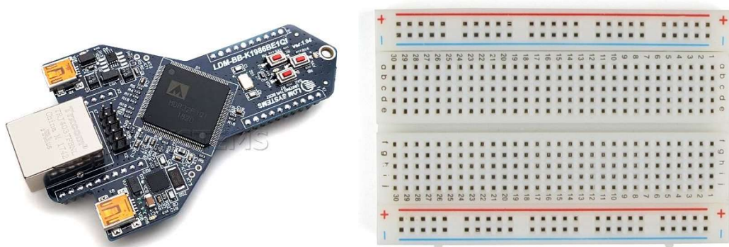
Рисунок 1. Общий вид отладочной платы LDM-BB-K1986BE1QI и панели типа Bread Board
