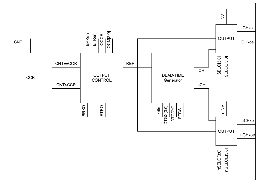
Рисунок 56 – Структурная схема блока сравнения
