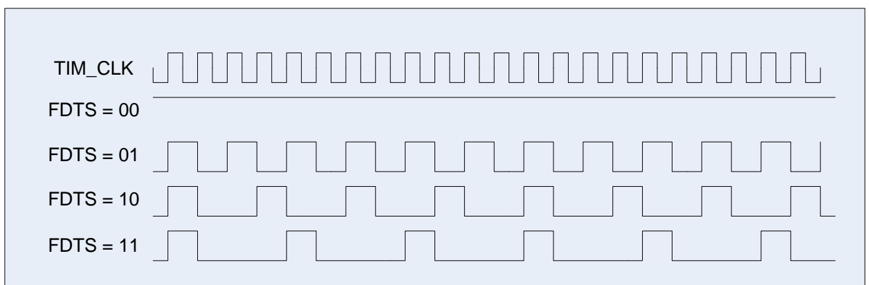
Рисунок 48 – Диаграммы возможных частот выборки данных (FDTs)
