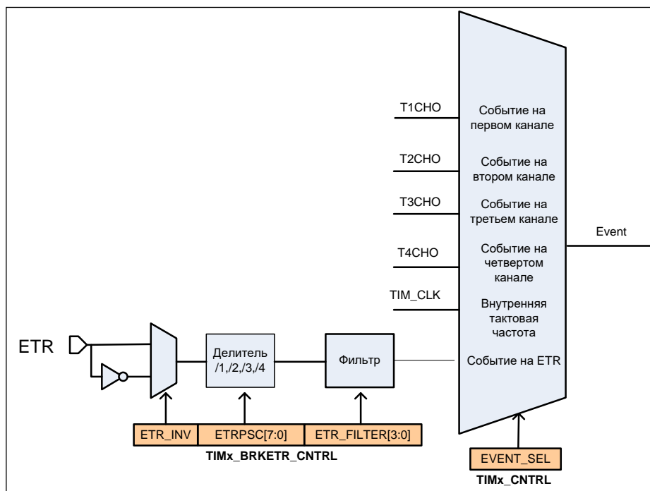
Рисунок 52 – Схема тактирования сигналом со входа ETR
