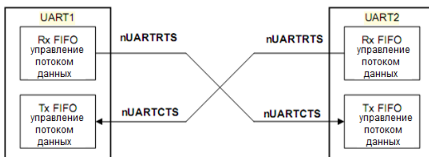
Рисунок 90 – Взаимодействие двух устройств последовательной связи с аппаратным управлением потоком данных
