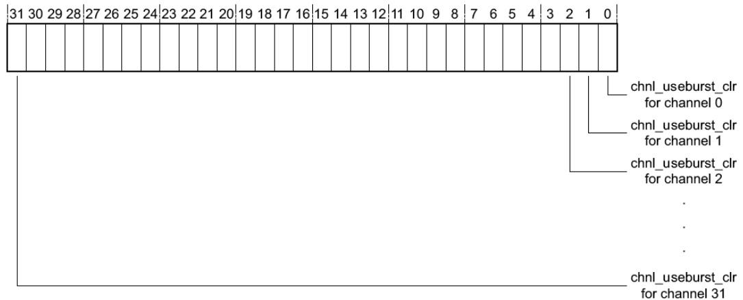
Рисунок 116 – Наименование разрядов регистра chnl_useburst_clr
