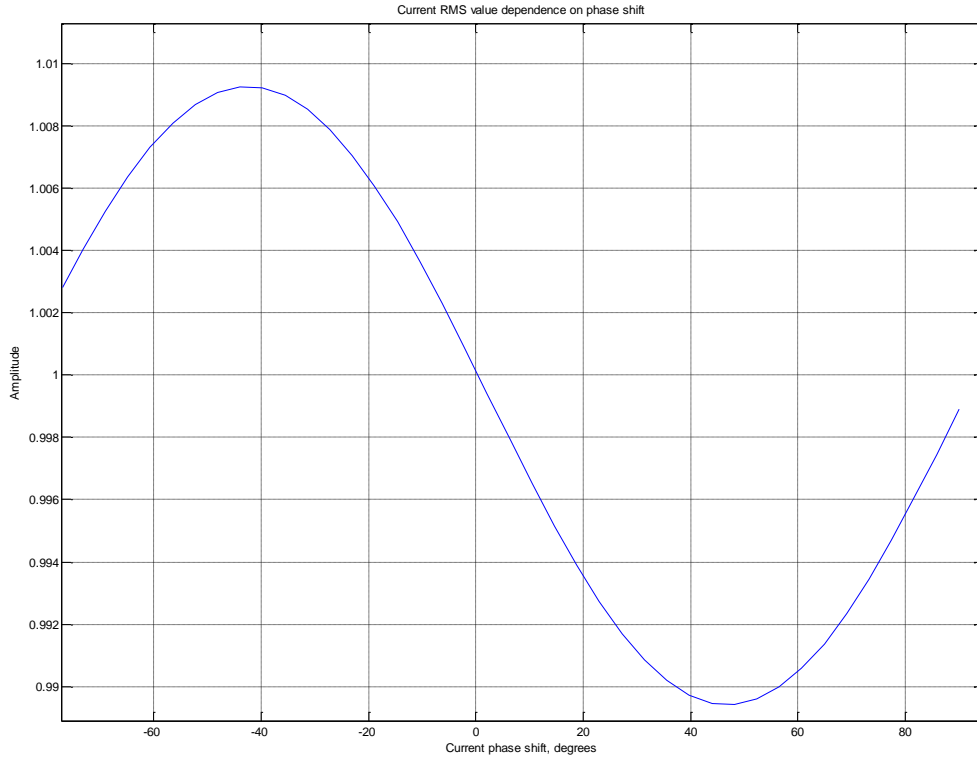
Рисунок 22 – Зависимость действующего значения тока от фазового сдвига
