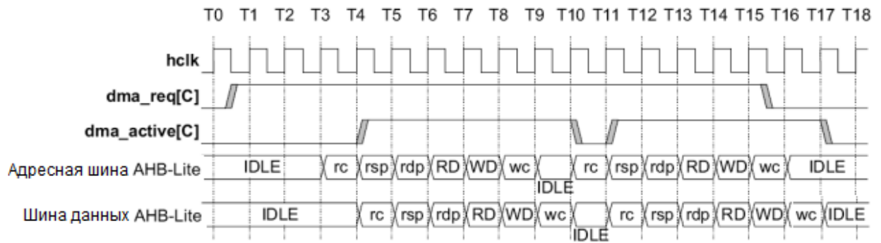
Рисунок 98 – Диаграмма работы при получении от периферийного блока запроса на обработку по уровню.
