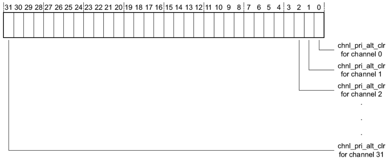
Рисунок 122 – Наименование разрядов регистра chnl_pri_alt_clr
