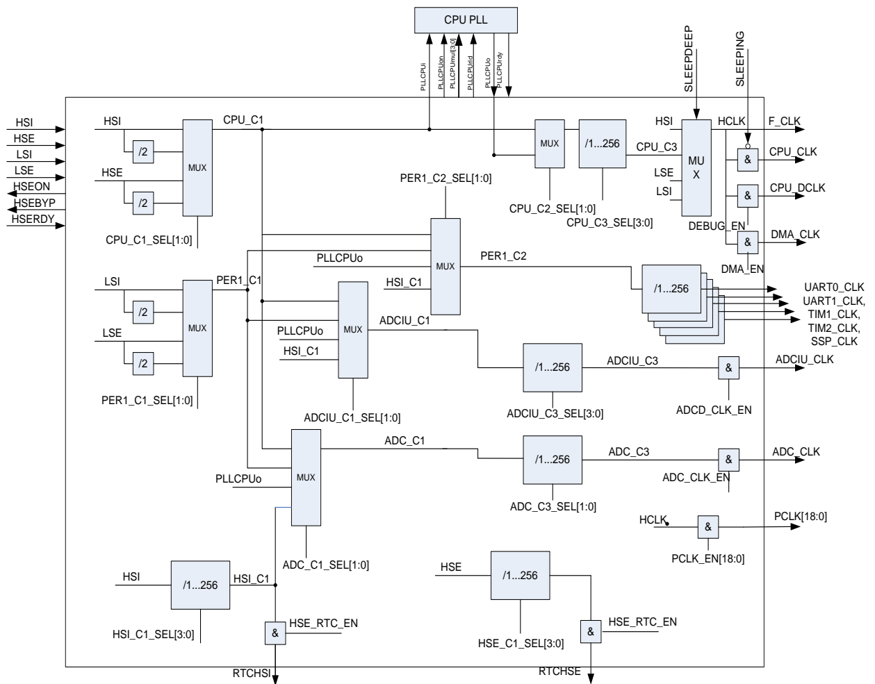
Рисунок 32 – Структурная схема
