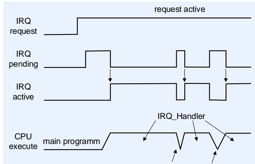
Рисунок 150 – Повторная обработка прерываний при удержании запроса от источника
