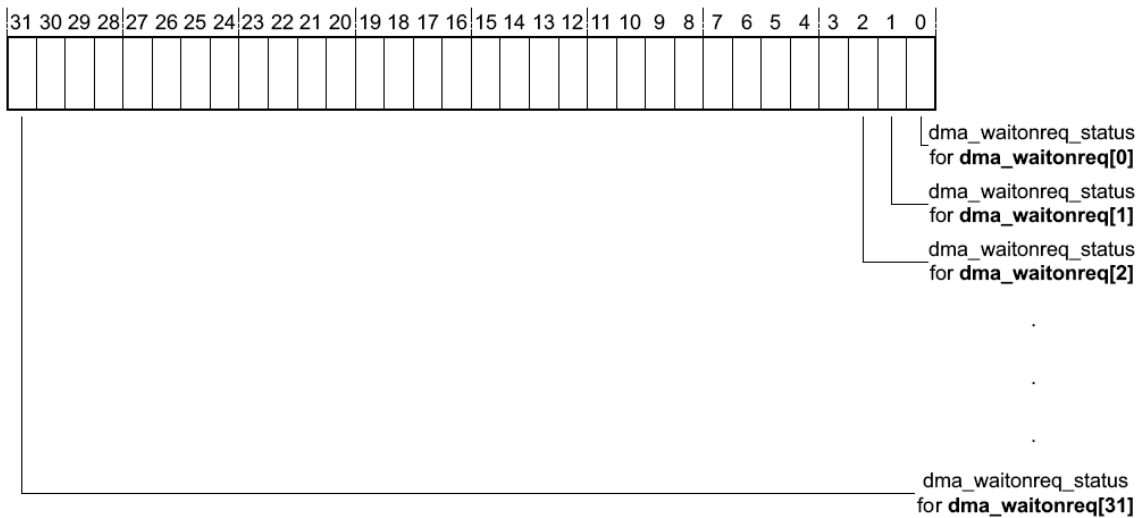
Рисунок 113 – Наименование разрядов регистра dma_waitonreq_status
