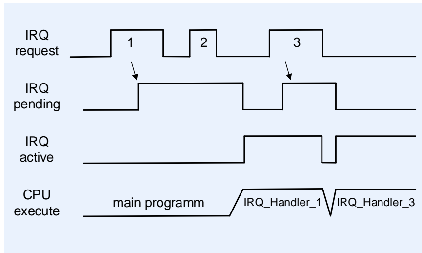
Рисунок 152 – Повторная установка запроса на прерывание в момент выполнения обработчика исключения
