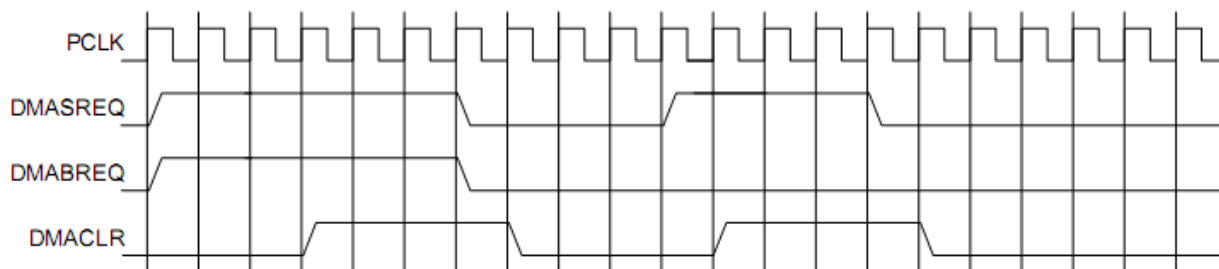
Рисунок 91 – Одноэлементный и блочный запросы ПДП
