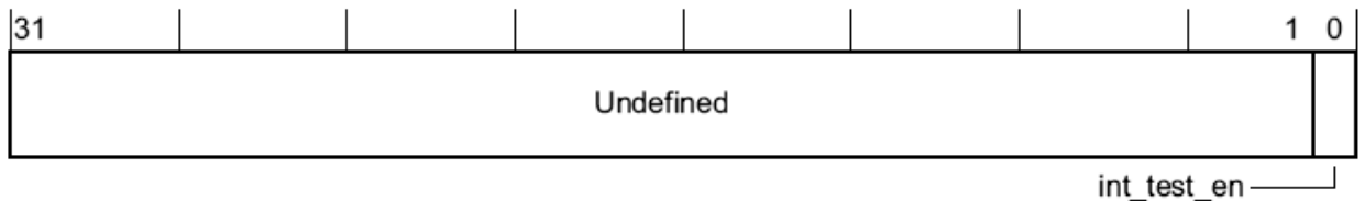
Рисунок 137 – Наименование разрядов регистра integration_cfg
