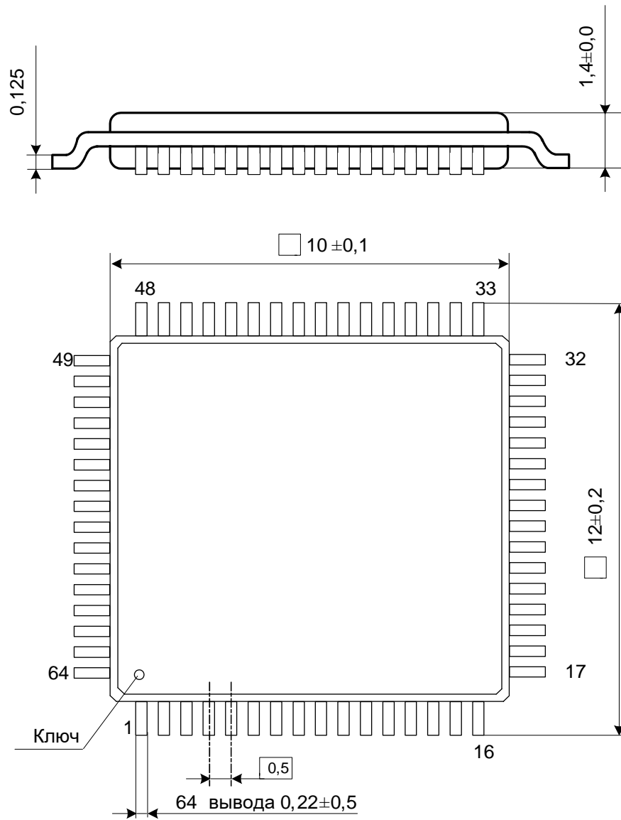
Рисунок 165 – Микросхема в корпусе LQFP64
