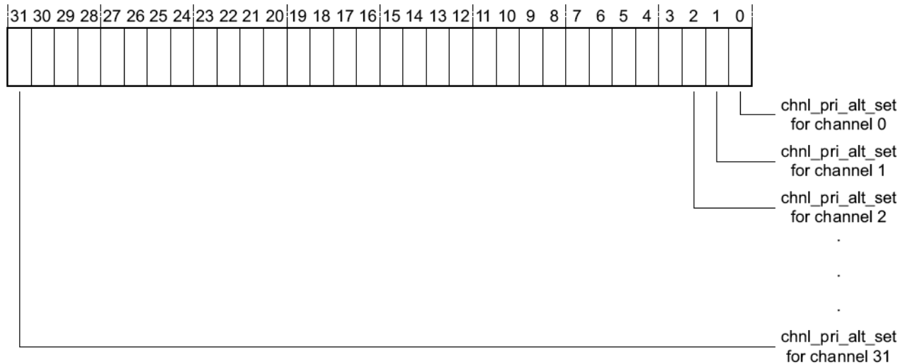
Рисунок 121 – Наименование разрядов регистра chnl_pri_alt_set
