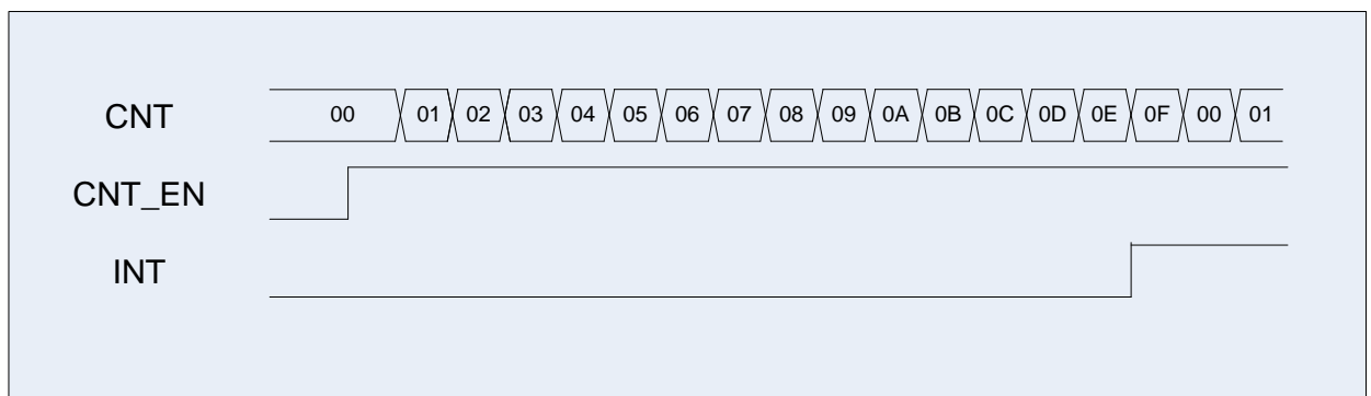
Рисунок 62 – Диаграммы примера работы в режиме обычного счетчика
