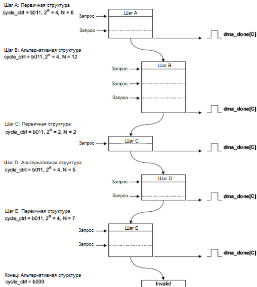
Рисунок 103 – Пример работы в режиме Пинг-понг
