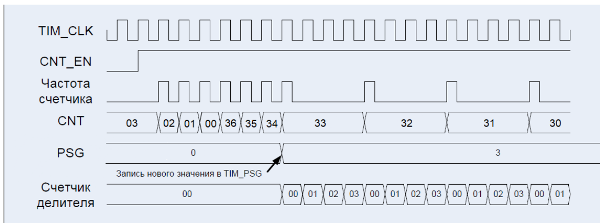
Рисунок 44 – Диаграммы работы счетчика: счет вниз (CNT_MODE = 00, EVENT_SEL = 0000, DIR = 1)
