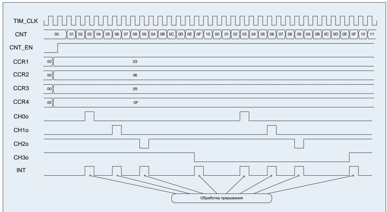
Рисунок 64 – Диаграммы примера работы в режиме ШИМ
