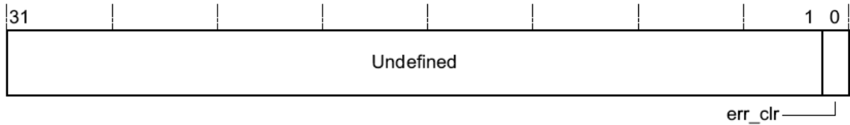
Рисунок 125 – Наименование разрядов регистра err_clr
