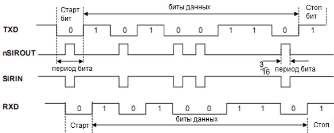
Рисунок 88 – Модуляция данных IrDA
