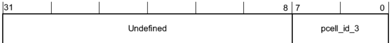
Рисунок 136 – Наименование разрядов регистра pcell_id_3
