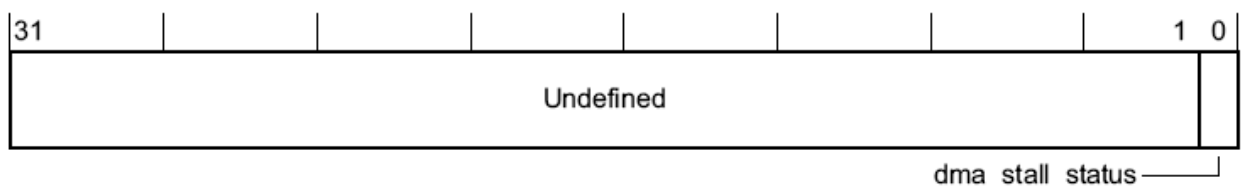
Рисунок 138 – Наименование разрядов регистра dma_stall_status
