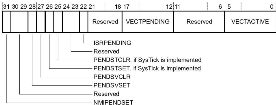
Рисунок 159 – Назначение разрядов регистра ICSR
