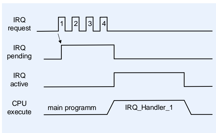
Рисунок 151 – Многократная установка снятие запроса IRQ request
