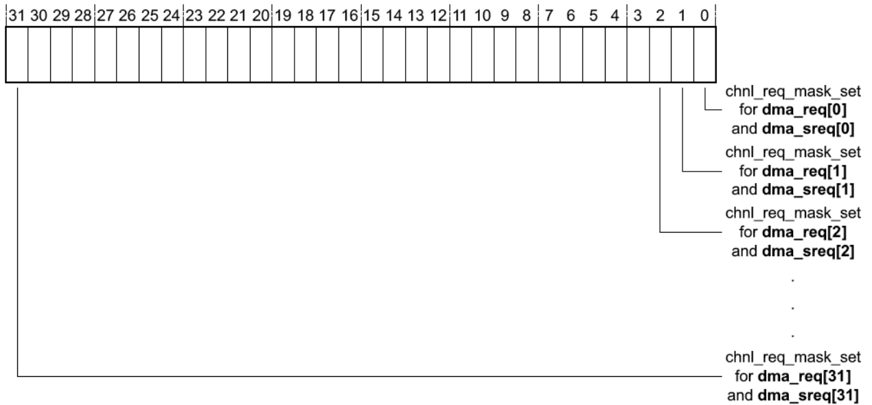
Рисунок 117 – Наименование разрядов регистра chnl_req_mask_set
