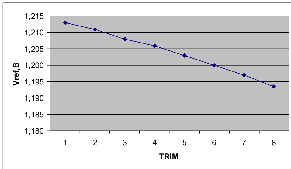
Рисунок 66 – Зависимость источника опорного напряжения от подстройки
