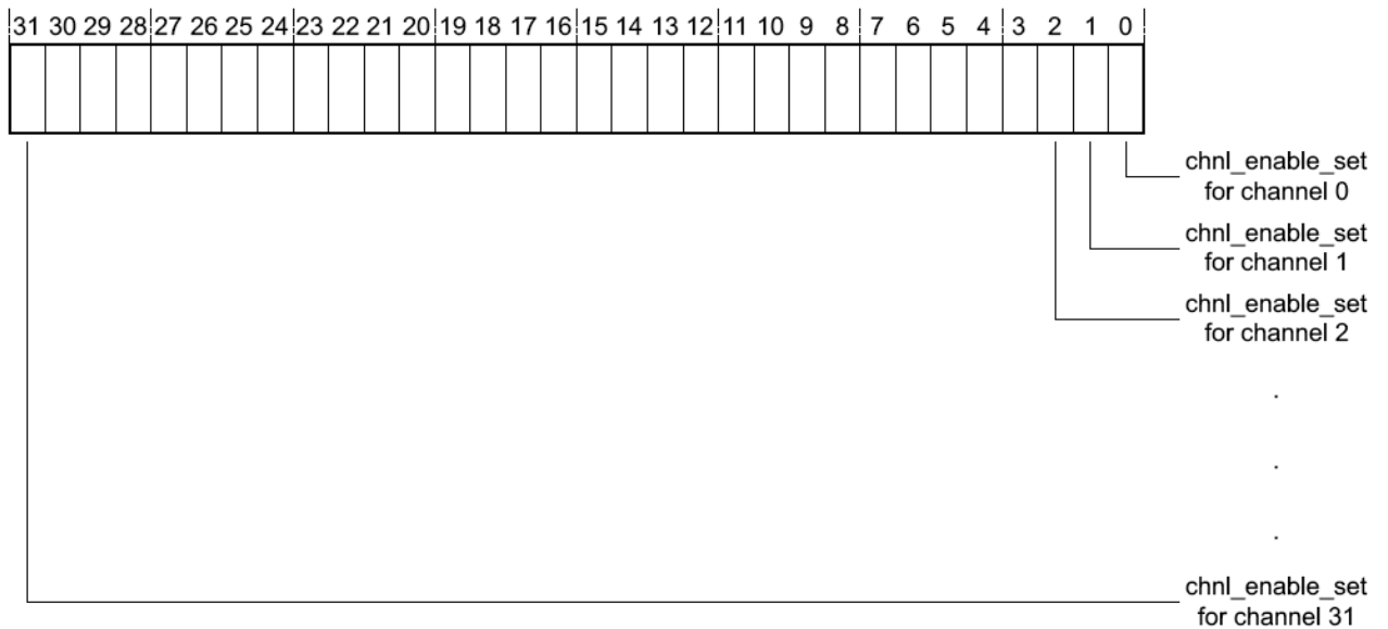
Рисунок 119 – Наименование разрядов регистра chnl_enable_set
