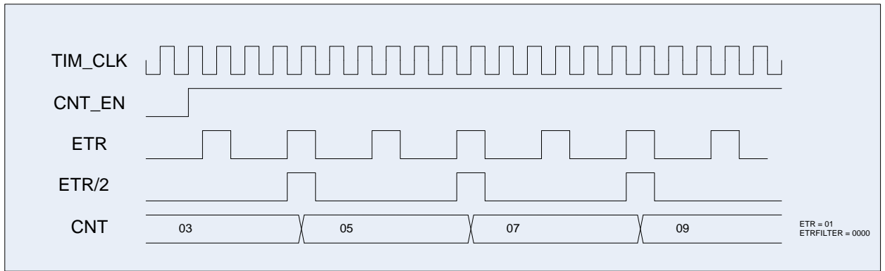
Рисунок 53 – Диаграмма тактирования сигналом со входа ETR
