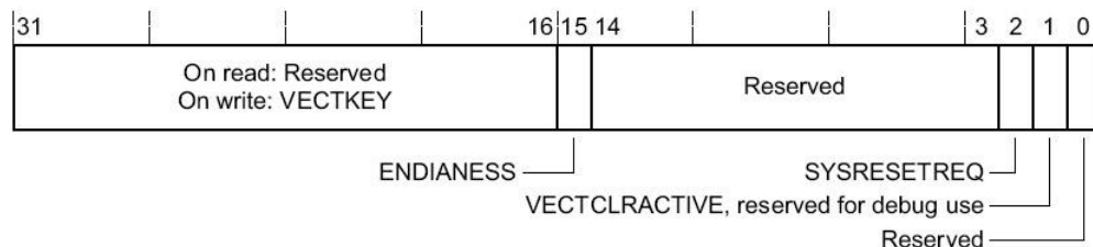
Рисунок 160 – Назначение разрядов регистра AIRCR
