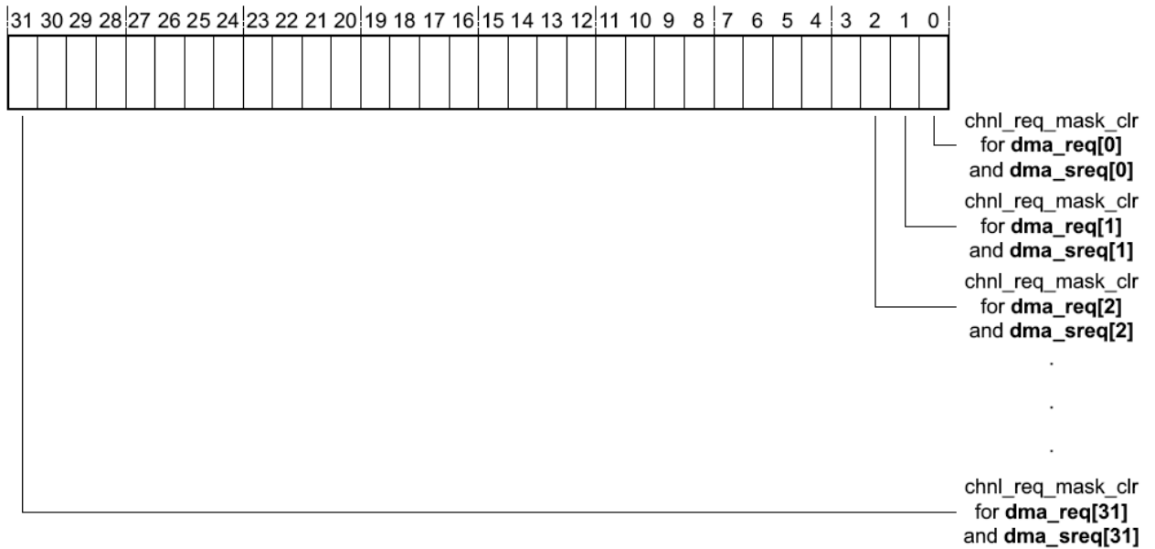
Рисунок 118 – Наименование разрядов регистра chnl_req_mask_clr
