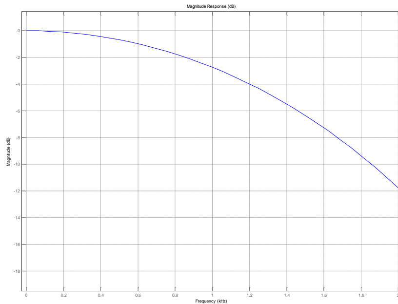
Рисунок 26 – Характеристика децимирующего фильтра в полосе 2 кГц
