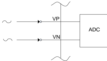
Рисунок 23 – Дифференциальное включение
