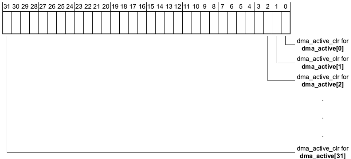
Рисунок 144 – Наименование разрядов регистра dma_active_clr
