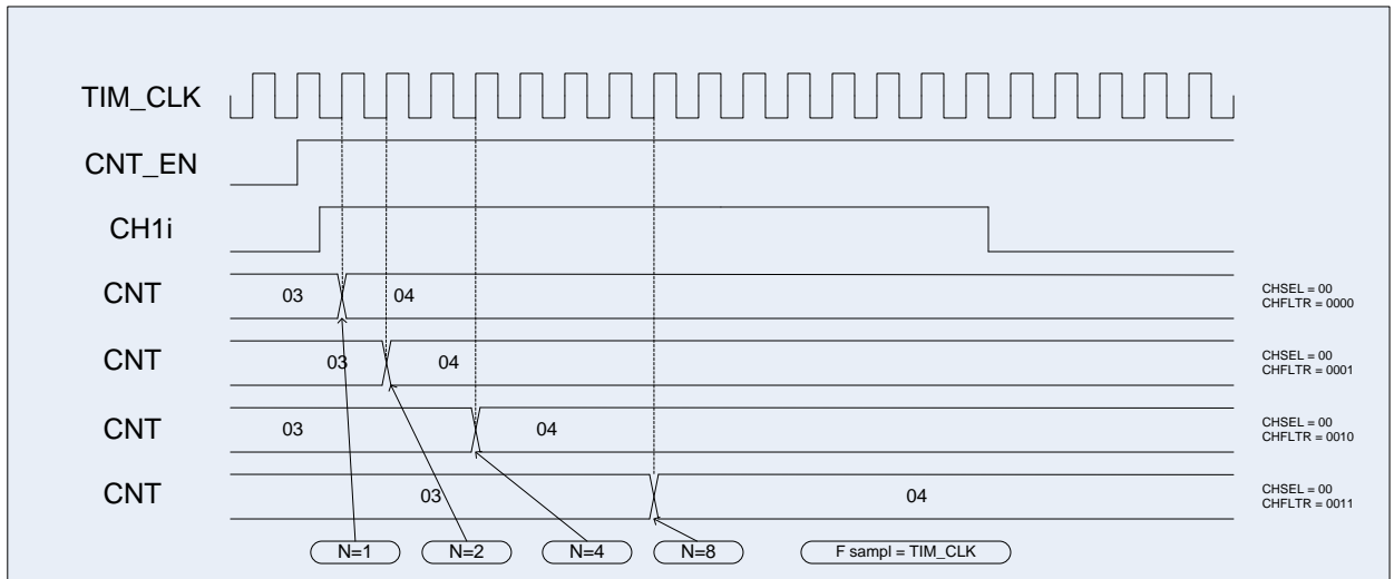
Рисунок 51 – Диаграмма внешнего тактирования с разными вариантами фильтра
