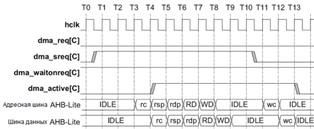
Рисунок 101 – Диаграмма работы контроллера ПДП при использовании периферией dma_waitonreq совместно с dma_sreq
