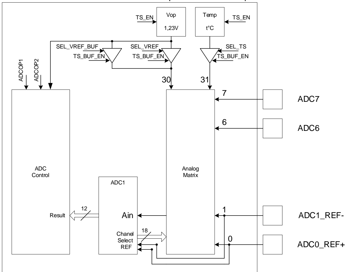
Рисунок 65 – Структурная схема контроллера АЦП
