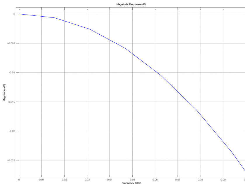
Рисунок 27 – Характеристика децимирующего фильтра в полосе 100 Гц
