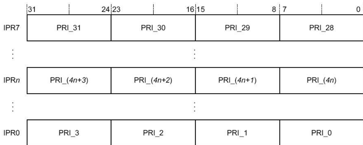
Рисунок 157 – Поля приоритета регистров IPR0-IPR7
