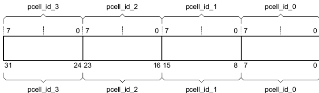
Рисунок 132 – Наименование разрядов регистра pcell_id_[3:0]
