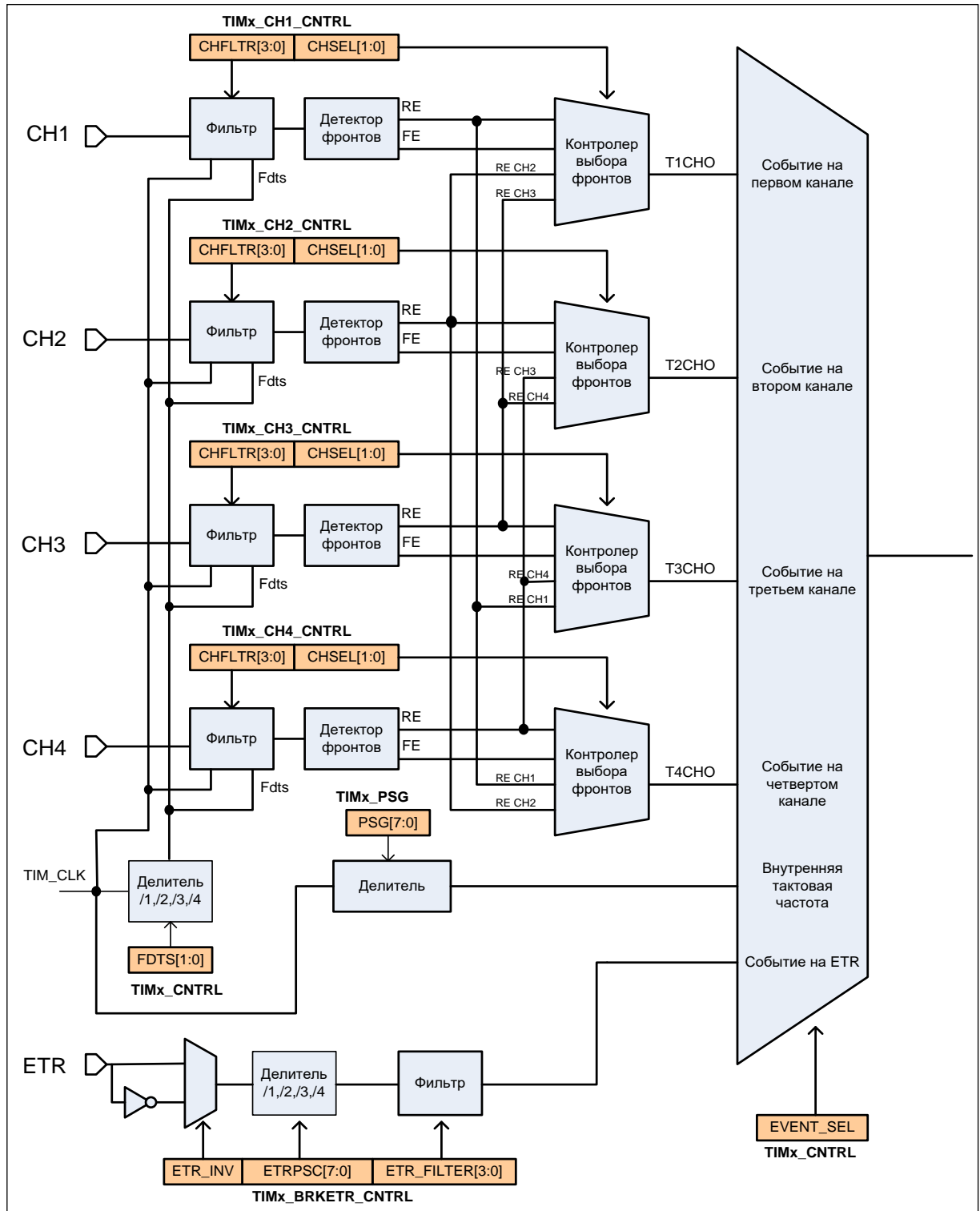
Рисунок 42 – Структурная схема формирования события для счета
