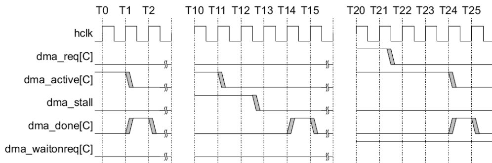
Рисунок 99 – Диаграммы функционирования dma_done
