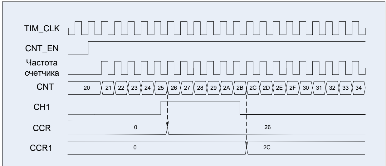
Рисунок 55 – Диаграмма захвата события со входа первого канала
