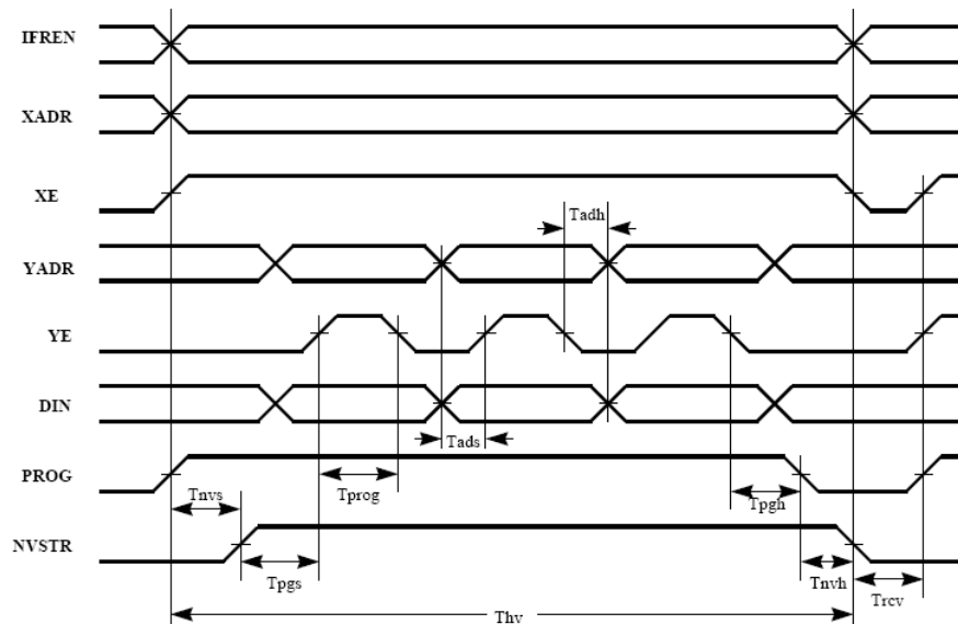
Рисунок 13 – Временная диаграмма записи памяти
