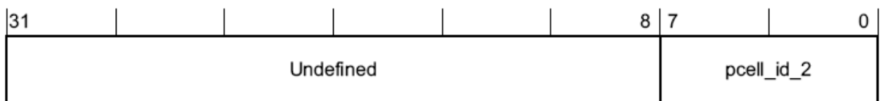
Рисунок 135 – Наименование разрядов регистра pcell_id_2
