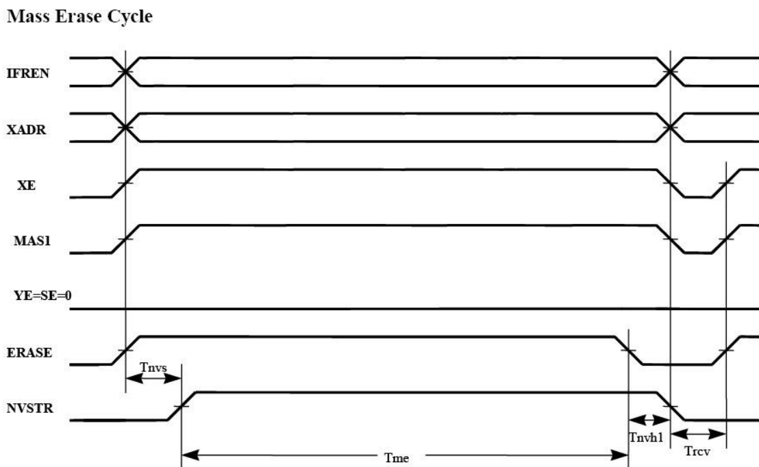
Рисунок 11 – Временная диаграмма стирания памяти
