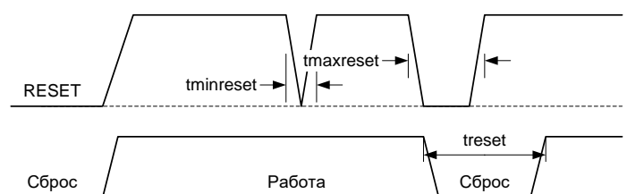
Рисунок 7 – Диаграмма фильтрации помех при формировании сброса
