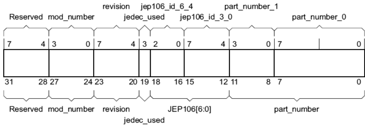
Рисунок 126 – Наименование разрядов регистров periph_id_[3:0]
