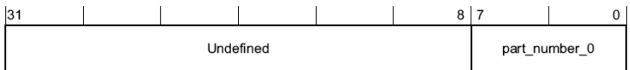
Рисунок 127 – Наименование разрядов регистра periph_id_0
