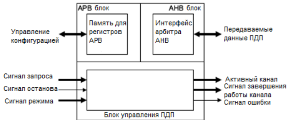
Рисунок 94 – Структурная схема контроллера
