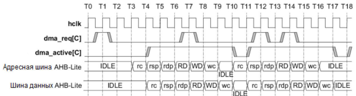
Рисунок 97 – Диаграмма работы при получении импульсного запроса от периферийного блока
