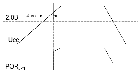
Рисунок 5 – Диаграмма формирования сброса микроконтроллера
