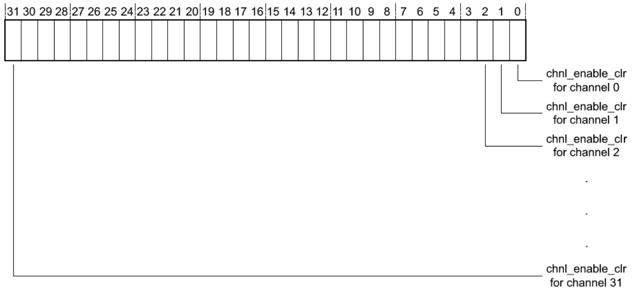
Рисунок 120 – Наименование разрядов регистра chnl_enable_clr
