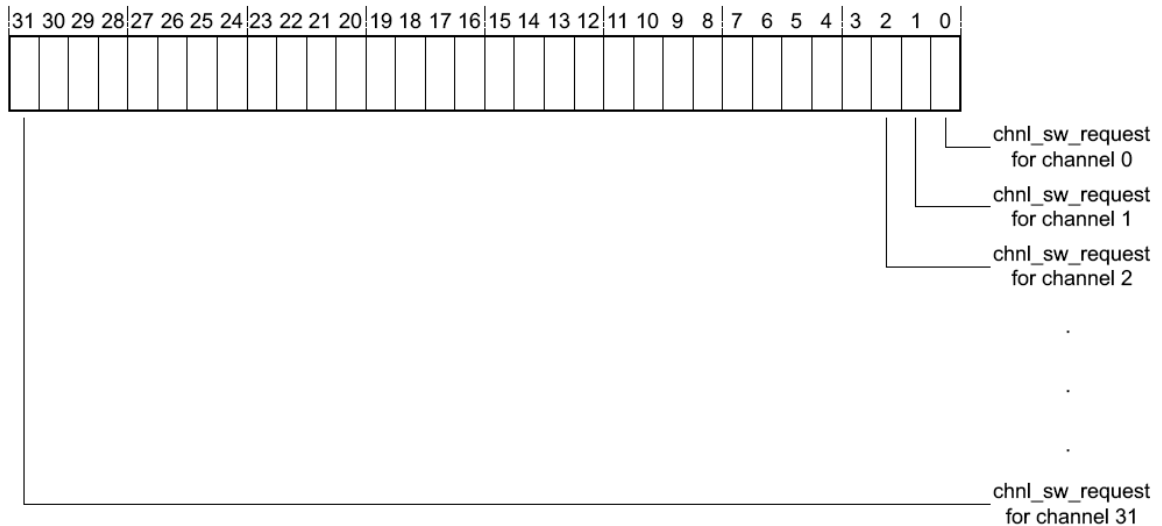
Рисунок 114 – Наименование разрядов регистра chnl_sw_request
