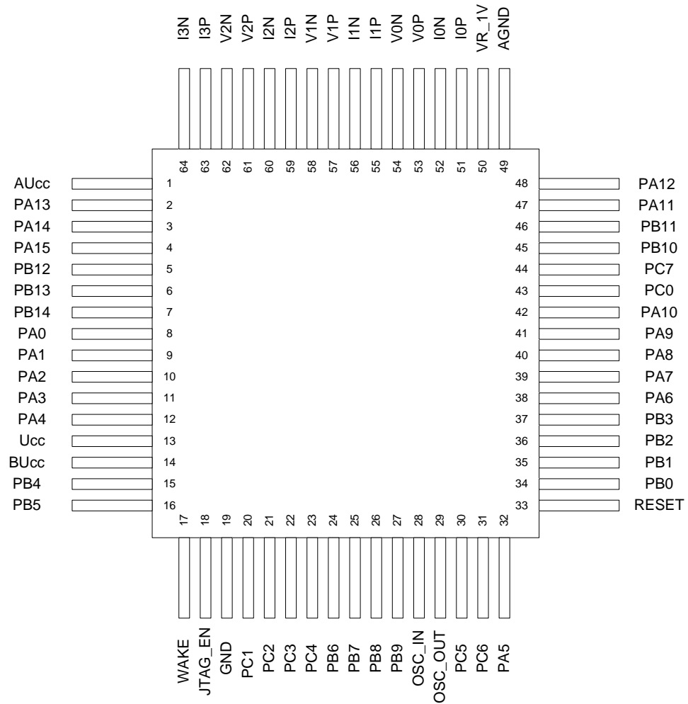
Рисунок 3 – Диаграмма расположения выводов
