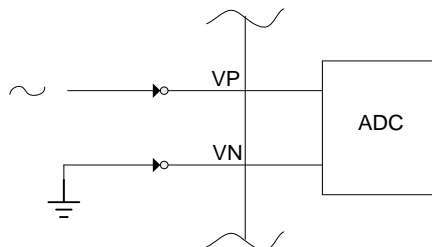
Рисунок 24 – Недифференциальное включение
