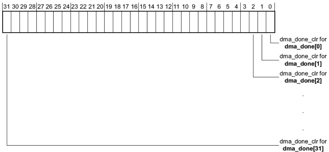
Рисунок 142 – Наименование разрядов регистра dma_done_clr
