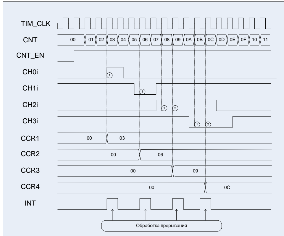
Рисунок 63 – Диаграммы примера работы в режиме захвата Режим ШИМ.
