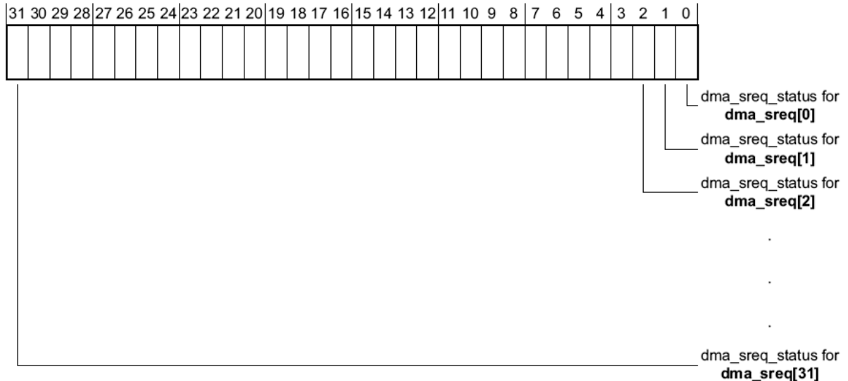
Рисунок 140 – Наименование разрядов регистра dma_sreq_status
