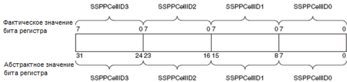
Рисунок 84 – Распределение бит в регистрах идентификации разработчика.
