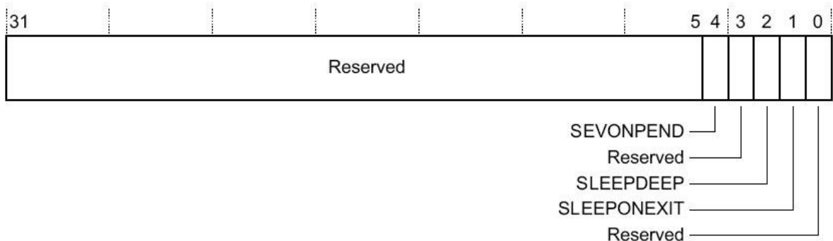
Рисунок 161 – Назначение разрядов регистра SCR
