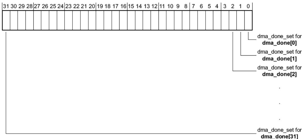
Рисунок 141 – Наименование разрядов регистра dma_done_set
