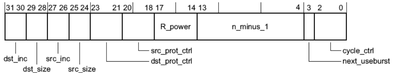
Рисунок 108 – Название разрядов channel_cfg
