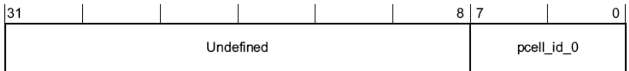
Рисунок 133 – Наименование разрядов регистра pcell_id_0
