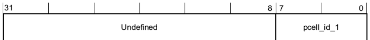
Рисунок 134 – Наименование разрядов регистра pcell_id_1
