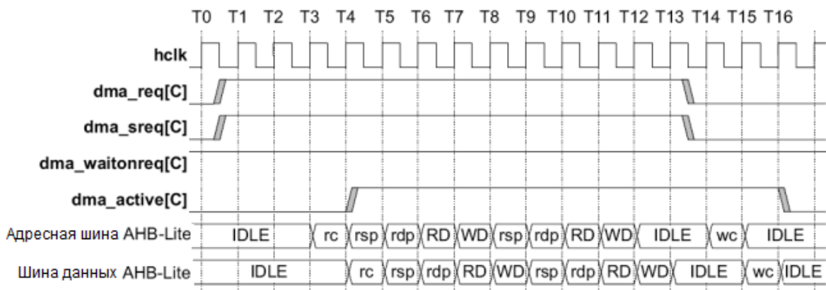
Рисунок 100 – Диаграмма работы контроллера ПДП при использовании периферией dma_waitonreq
