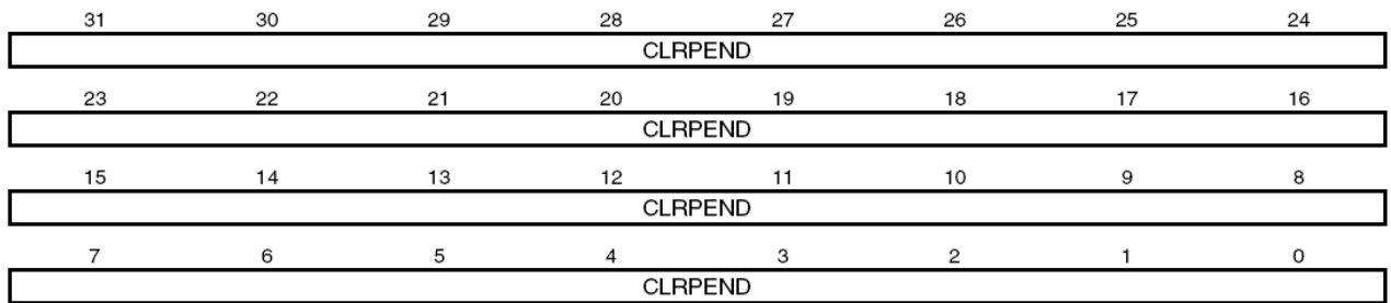
Рисунок 156 – Распределение бит регистра ICPR
