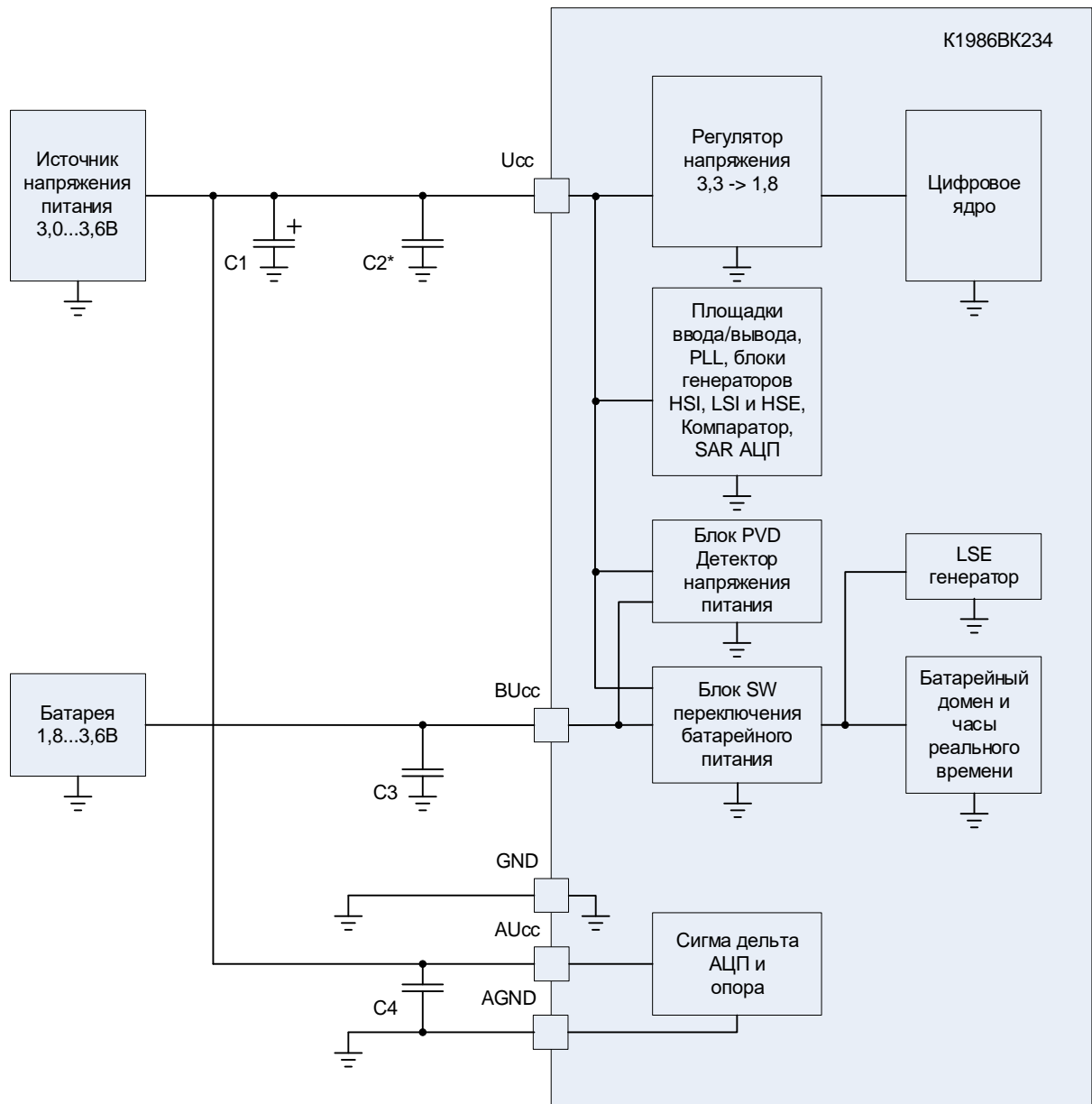
Рисунок 4 – Структурная схема подачи питания
