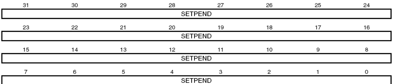
Рисунок 155 – Распределение бит регистра ISPR
