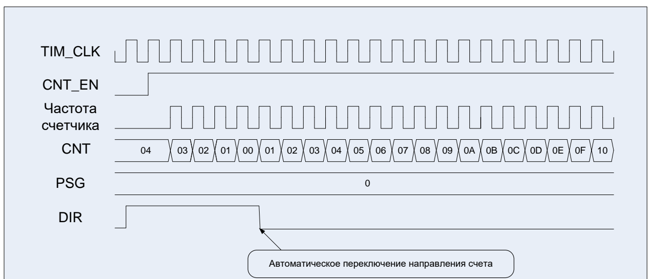
Рисунок 41 – Диаграммы работы таймера, счет вверх/вниз, сначала вниз
