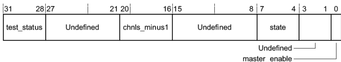
Рисунок 109 – Наименование разрядов регистра dma_status
