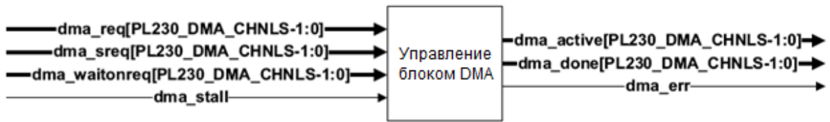
Рисунок 95 – Сигналы интерфейса управления ПДП
