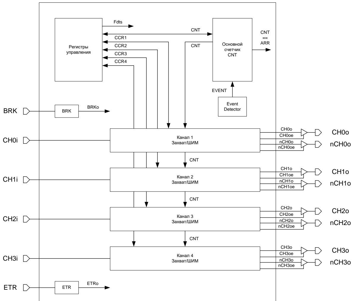
Рисунок 37 – Структурная схема таймера
