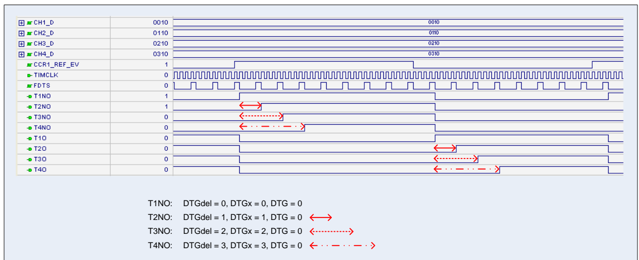
Рисунок 60 – Диаграмма работы схемы DTG
