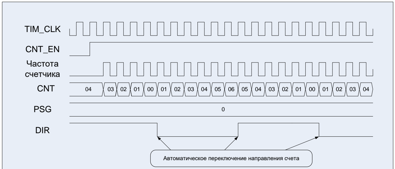
Рисунок 45 – Диаграммы работы счетчика: счет вниз/вверх (CNT_MODE = 01, EVENT_SEL = 0000, DIR = 1)
