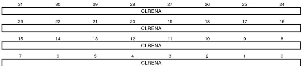
Рисунок 154 – Распределение бит регистра ICER
