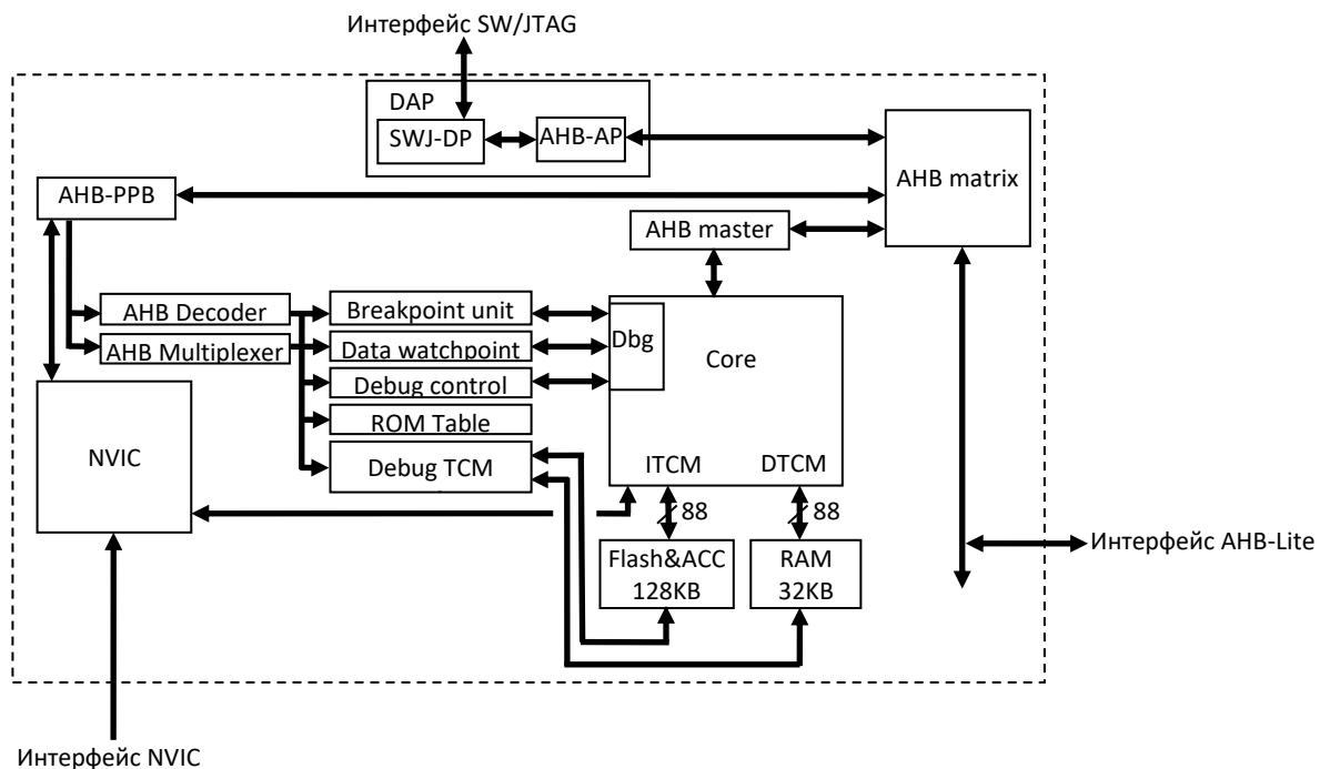
Рисунок 15 – Структурная схема процессора
