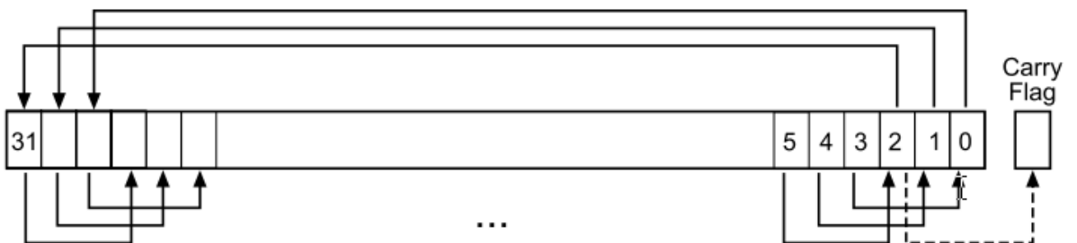
Рисунок 20 – Инструкция ROR # 3
