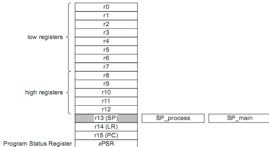
Рисунок 16 – Регистры ядра
