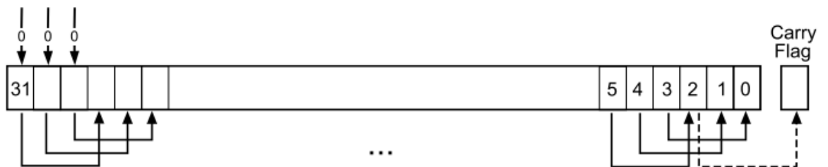
Рисунок 18 – Инструкция LSR # 3
