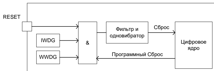
Рисунок 6 – Блок-схема формирования сброса микроконтроллера
