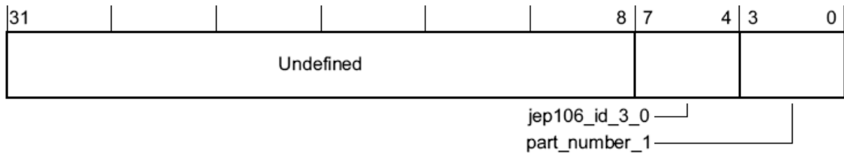
Рисунок 128 – Наименование разрядов регистра periph_id_1
