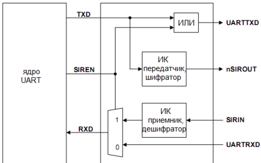
Рисунок 86 – Структурная схема кодека
