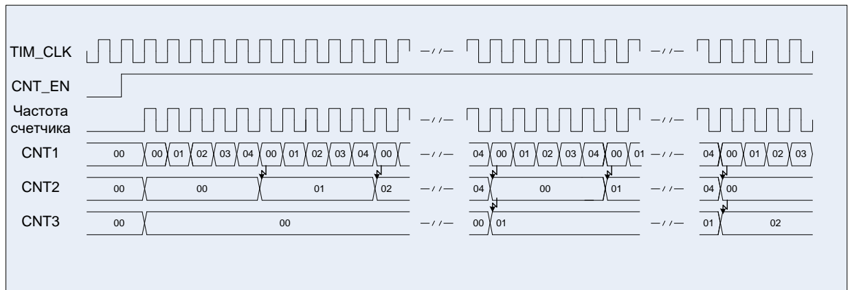
Рисунок 47 – Диаграммы работы трех таймеров в каскаде
