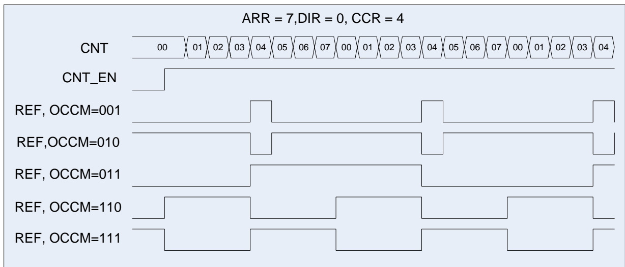
Рисунок 58 – Диаграмма работы схемы в режиме ШИМ, CCR1_EN=0
