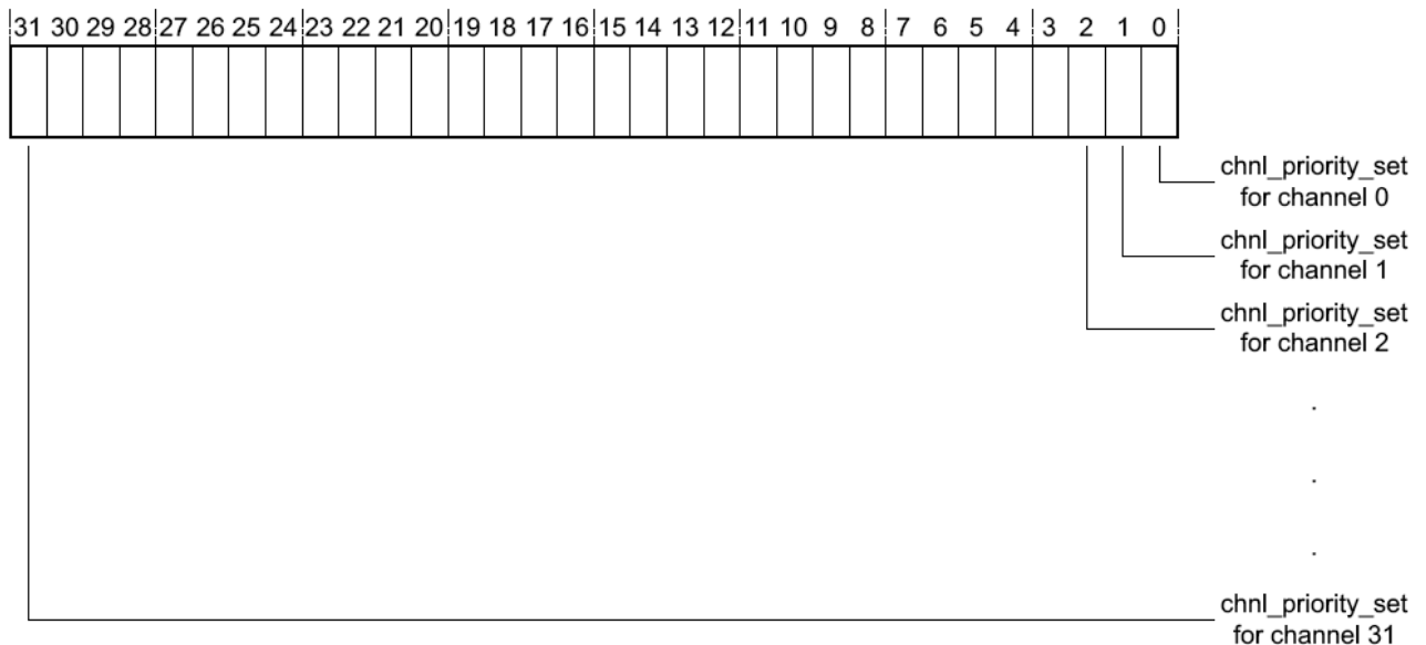
Рисунок 123 – Наименование разрядов регистра chnl_priority_set
