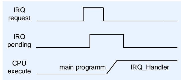
Рисунок 147 – Выставление отложенного запроса на прерывание и последующая его обработка
