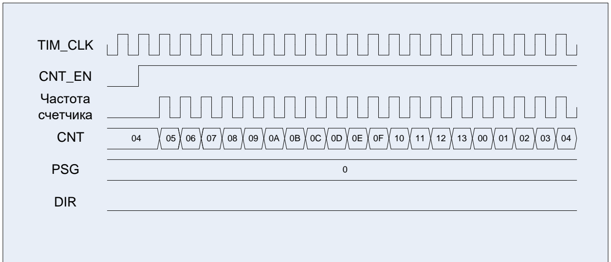
Рисунок 38 – Диаграммы работы таймера, счет вверх от 0 до 0x0013, стартовое значение 0x0004
