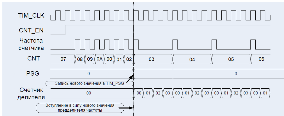
Рисунок 43 – Диаграммы работы счетчика: счет вверх (CNT_MODE = 00, EVENT_SEL = 0000, DIR = 0)
