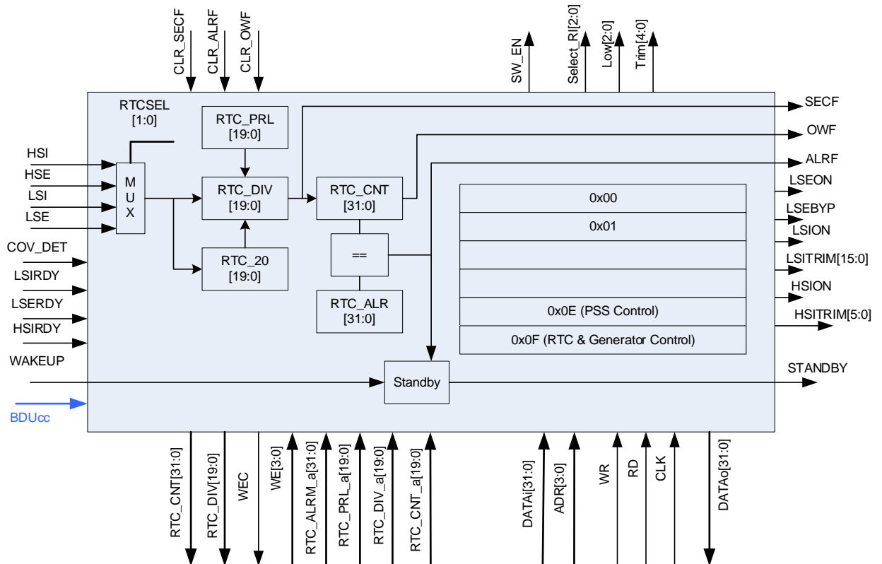
Рисунок 33 – Структурная схема
