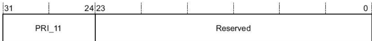
Рисунок 163 – Назначение разрядов регистра №2
