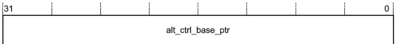
Рисунок 112 – Наименование разрядов регистра alt_ctrl_base_ptr
