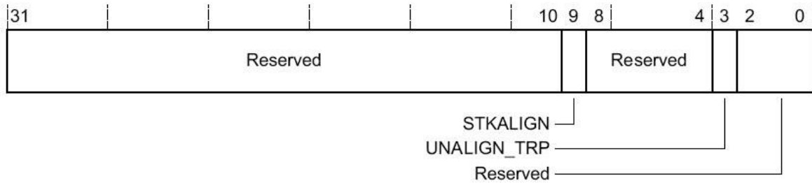
Рисунок 162 – Назначение разрядов регистра CCR
