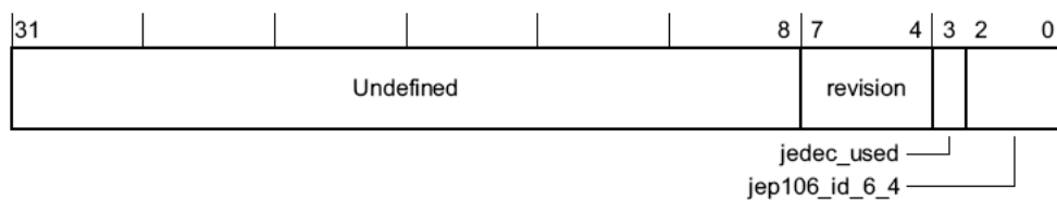
Рисунок 129 – Наименование разрядов регистра periph_id_2
