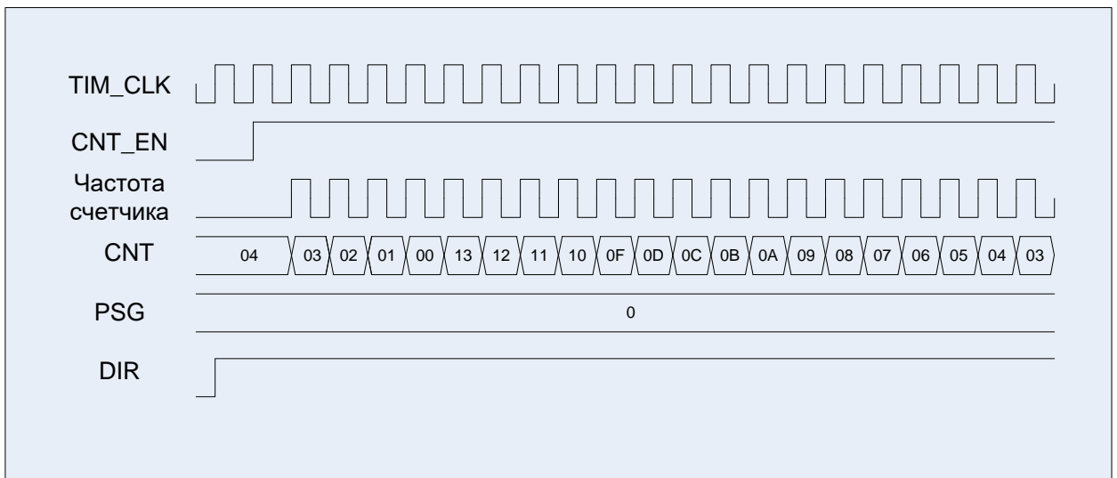
Рисунок 39 – Диаграммы работы таймера, счет вниз от 0x0013 до 0, стартовое значение 0x0004
