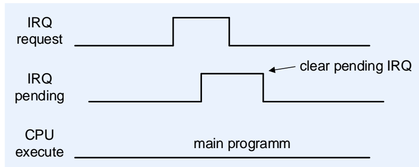
Рисунок 148 – Сброс признака отложенного прерывания, до обработки ядром
