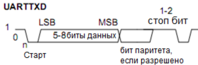
Рисунок 89 – Кадр передачи данных
