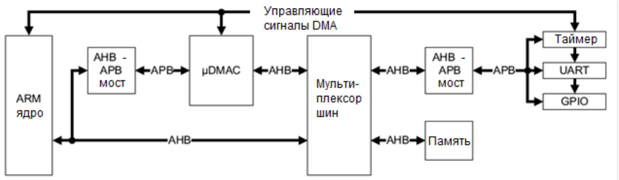
Рисунок 96 – Пример структурной схемы микроконтроллера с использованием контроллера ПДП
