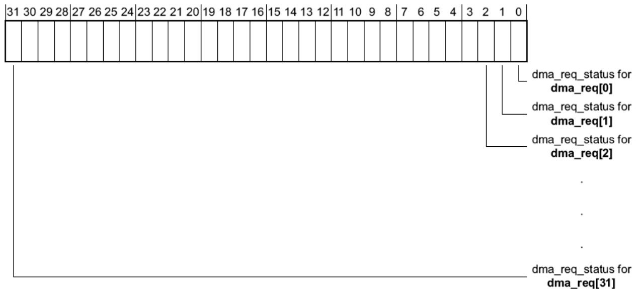
Рисунок 139 – Наименование разрядов регистра dma_req_status
