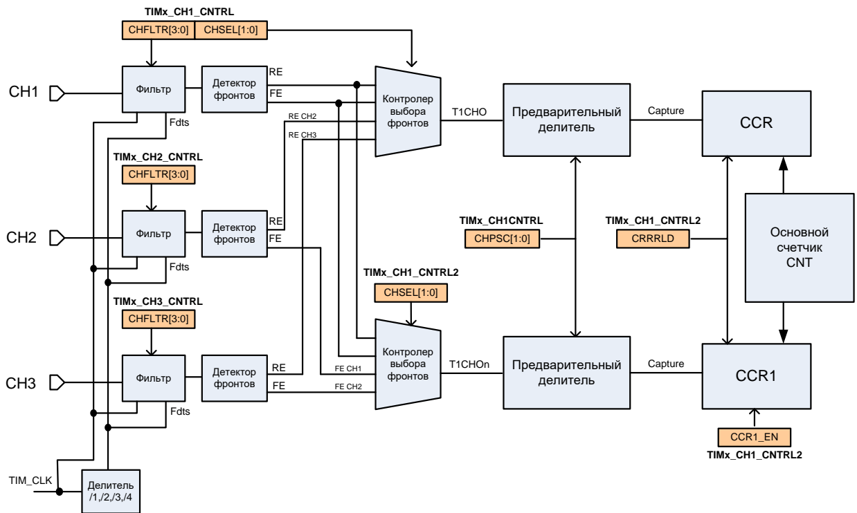
Рисунок 54 – Структурная схема блока захвата на примере канала 1
