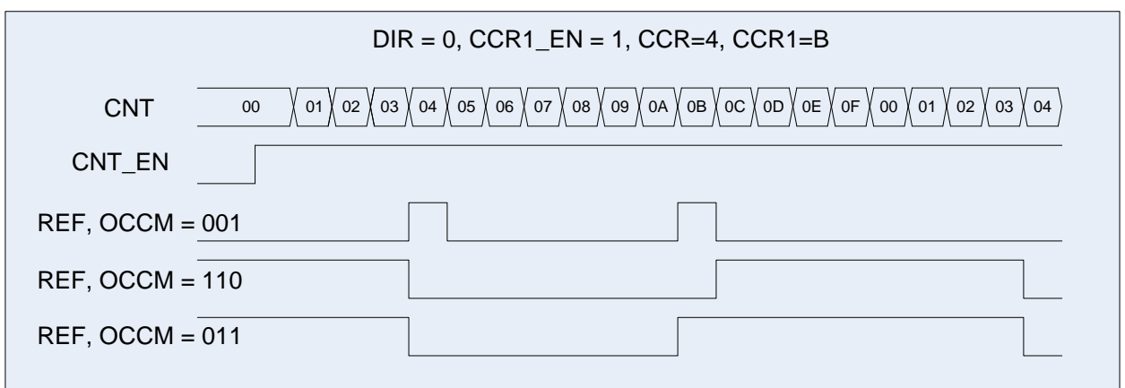
Рисунок 61 – Диаграмма работы схемы в режиме ШИМ, CCR1_EN = 1
