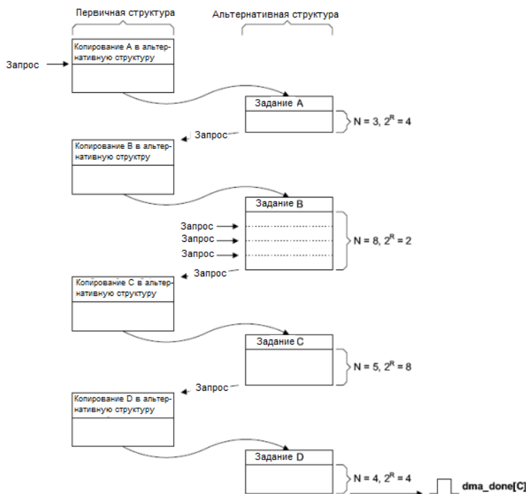
Рисунок 105 – Пример функционирования контроллера в режиме работы с периферией «исполнение с изменением конфигурации»
