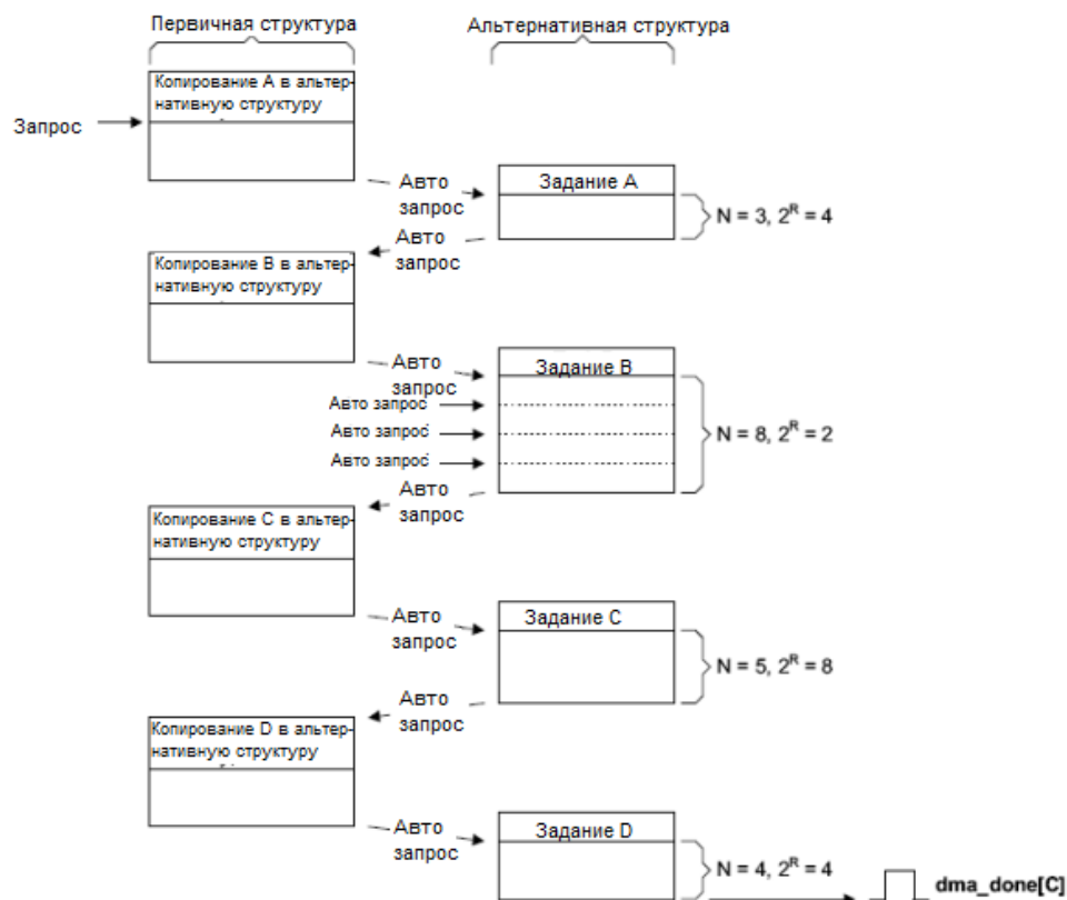
Рисунок 104 – Пример функционирования контроллера в режиме работы с памятью «исполнение с изменением конфигурации»
