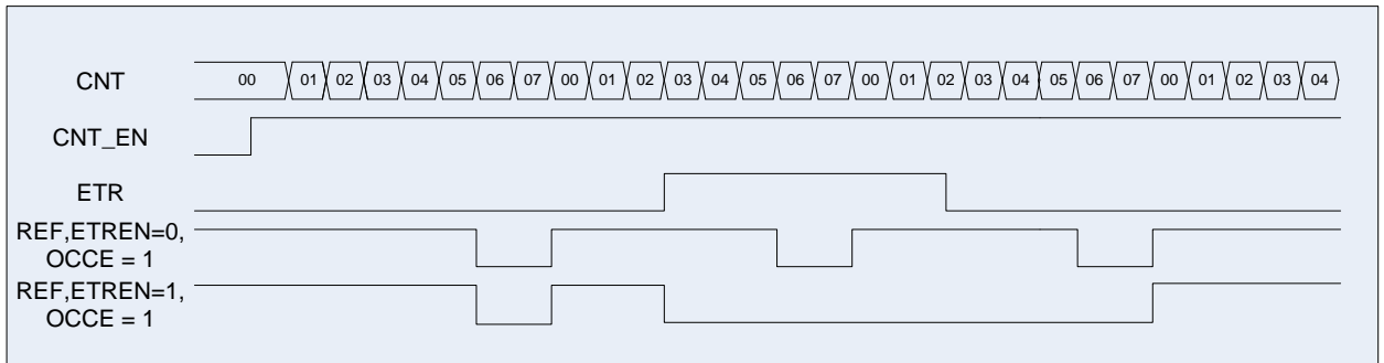
Рисунок 59 – Диаграмма работы схемы в режиме ШИМ, CCR1_EN = 0
