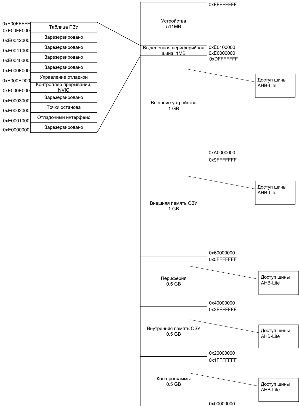
Рисунок 9 – Структура адресного пространства микроконтроллера
