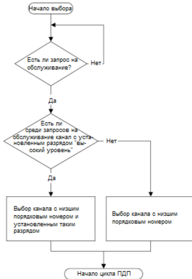
Рисунок 102 – Алгоритм выбора следующего канала для обслуживания.
