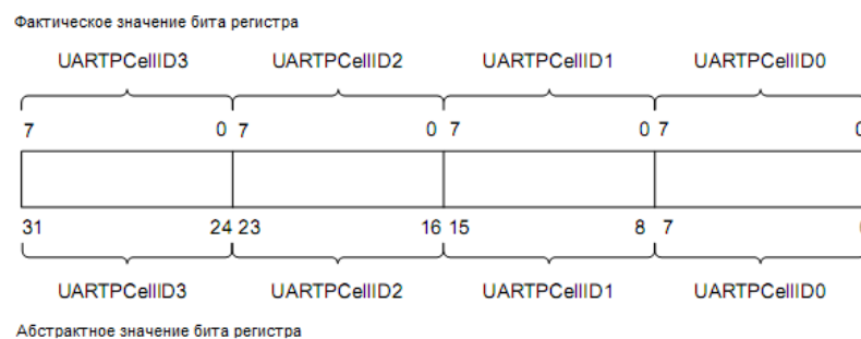
Рисунок 93 – Распределение бит в регистрах UARTPCellID0-3
