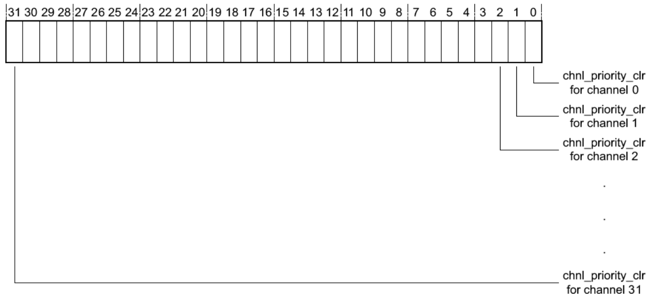
Рисунок 124 – Наименование разрядов регистра chnl_priority_clr
