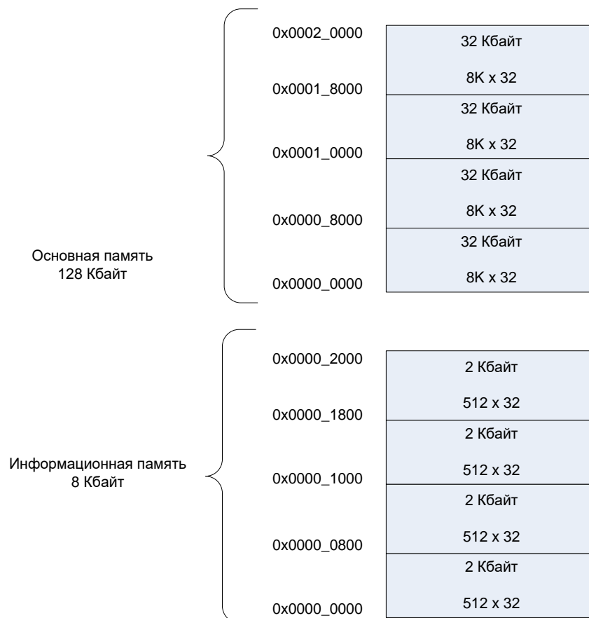
Рисунок 10 – Структура памяти
