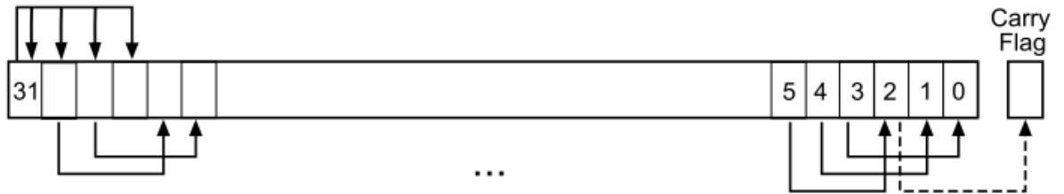
Рисунок 17 – Инструкция ASR # 3
