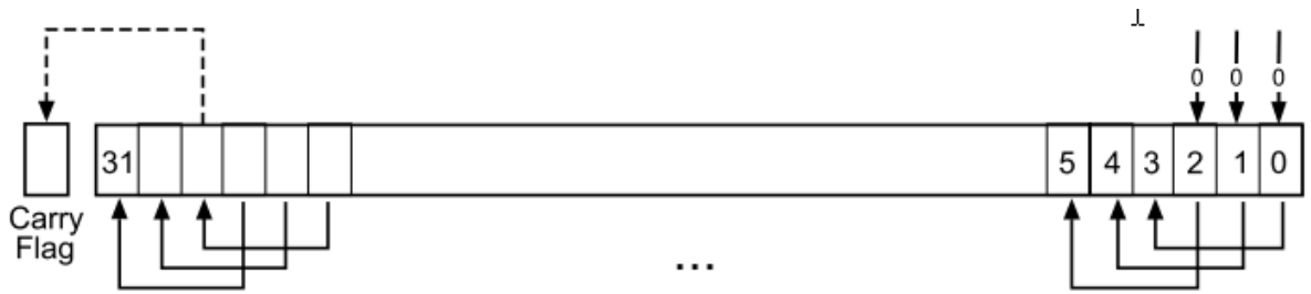
Рисунок 19 – Инструкция LSL # 3
