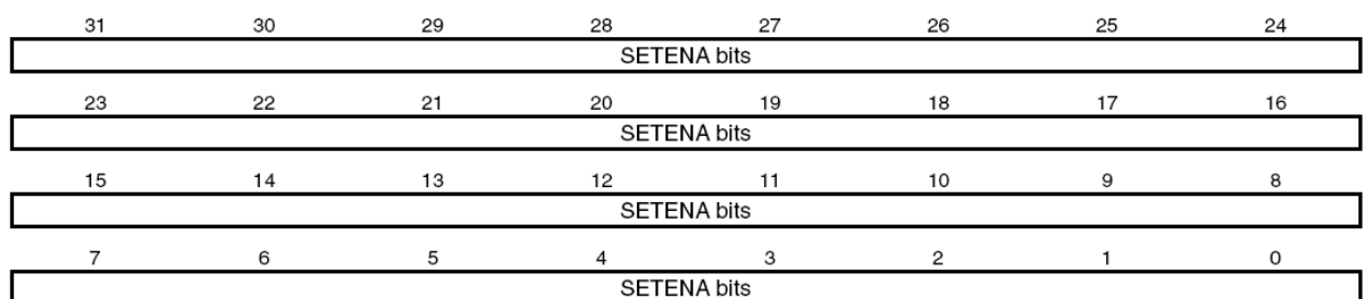
Рисунок 153 – Распределение бит регистра ISER
