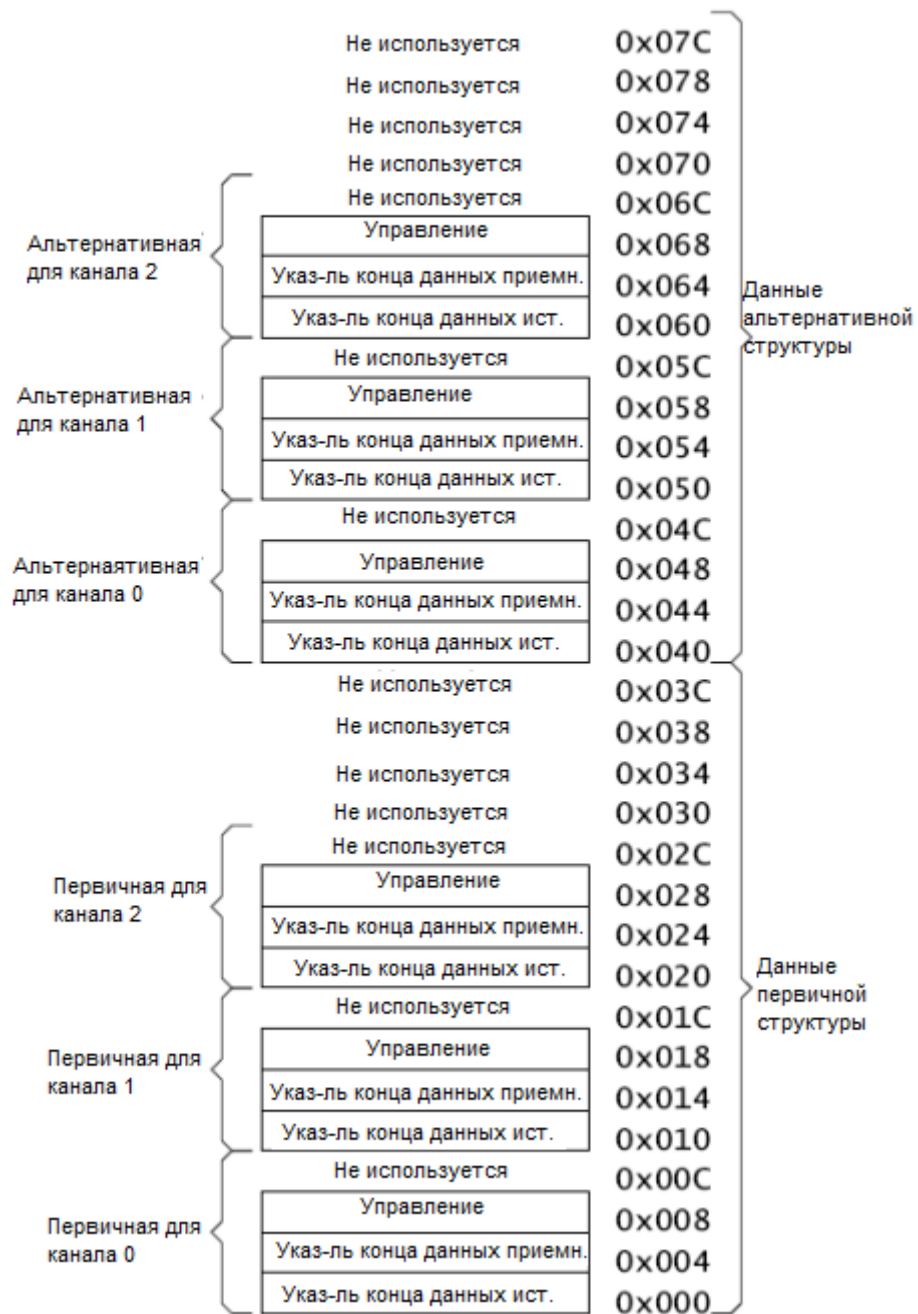
Рисунок 107 – Карта памяти для трех каналов ПДП, включая альтернативную структуру управляющих данных
