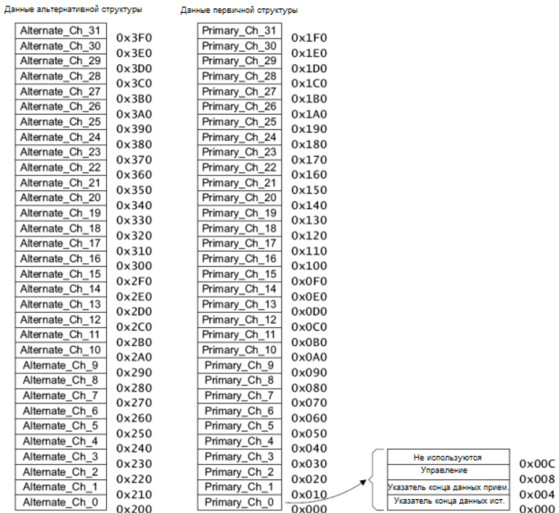
Рисунок 106 – Карта памяти для 32-х каналов, включая альтернативную структуру управляющих данных
