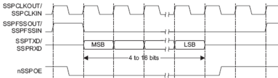
Рисунок 68 – Формат синхронного обмена протокола SSI фирмы Texas Instruments (единичный обмен)
