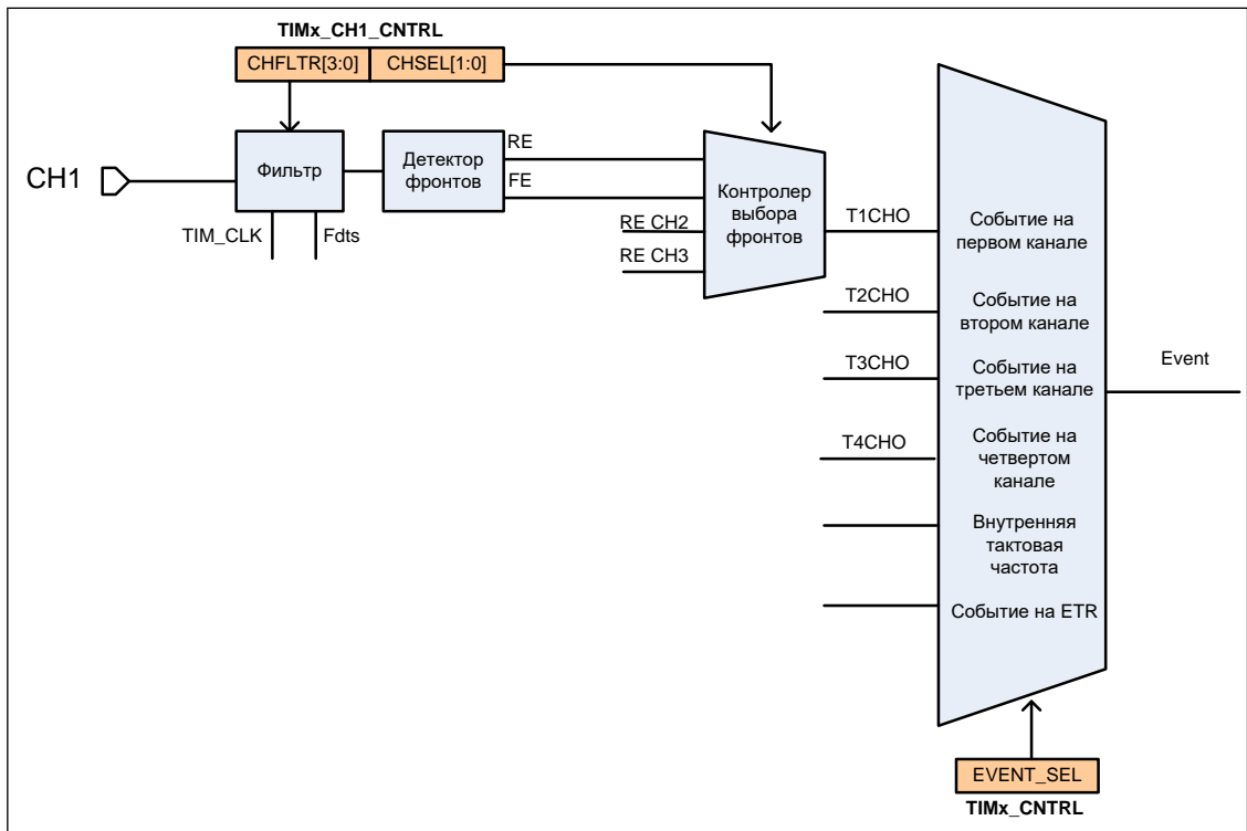
Рисунок 49 – Тактирование с входа первого канала
