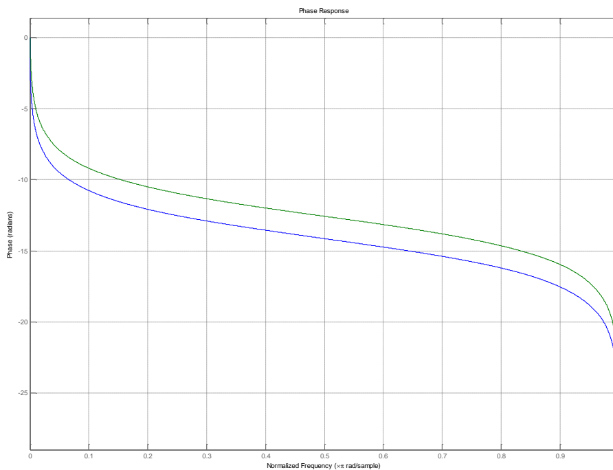
Рисунок 28 – Фильтр для сдвига сигнала на 90 градусов
