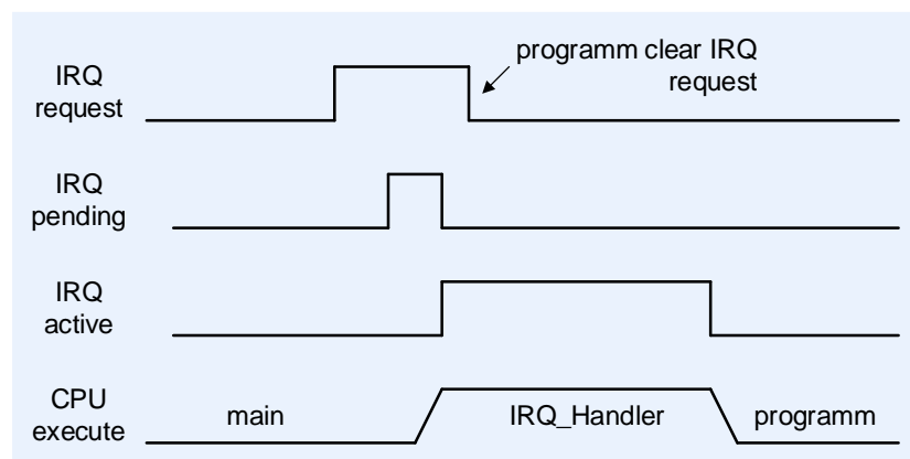
Рисунок 149 – Сброс признака отложенного прерывания, до обработки ядром
