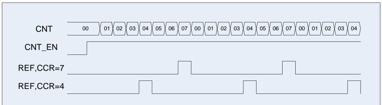
Рисунок 57 – Диаграмма работы схемы в режиме ШИМ, CCR1_EN=0
