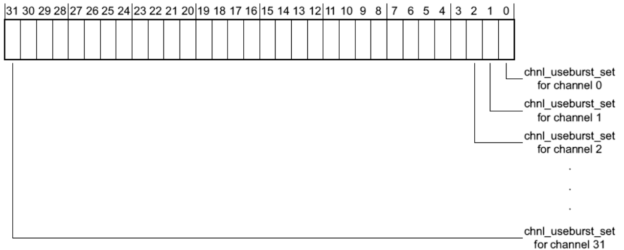
Рисунок 115 – Наименование разрядов регистра chnl_useburst_set
