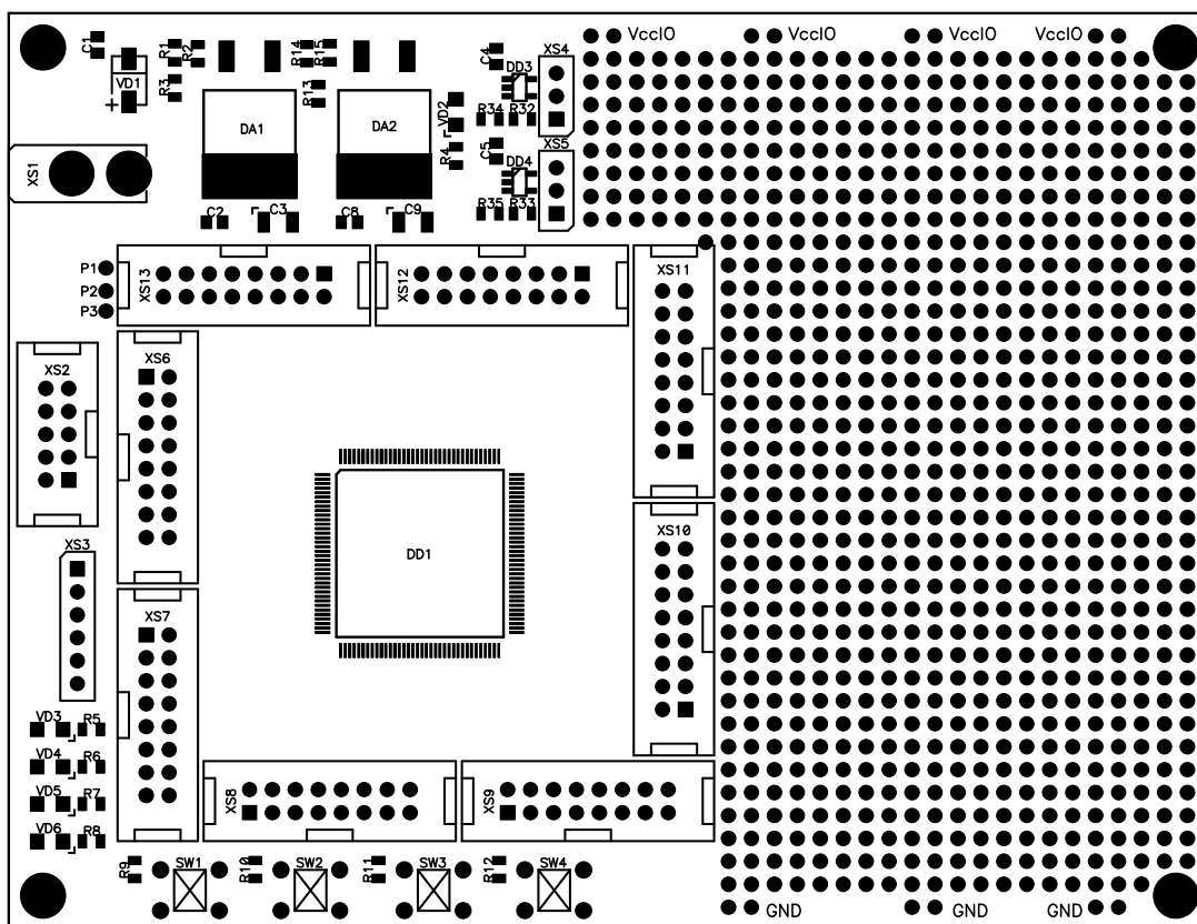
Рис. 5. Внешний вид печатной платы
